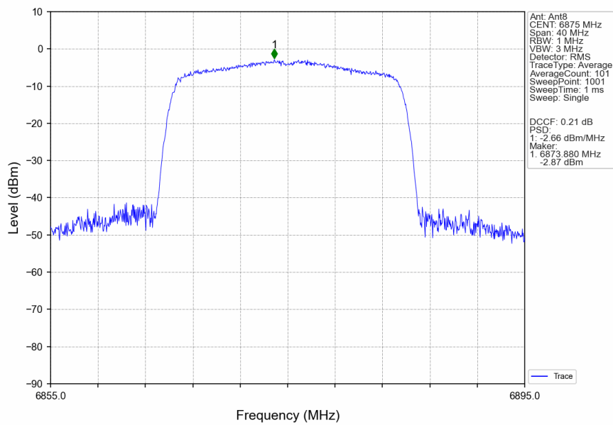
802.11be(EHT20)_HCH_6875MHz_RU242_Left_Ant8_NTNV
