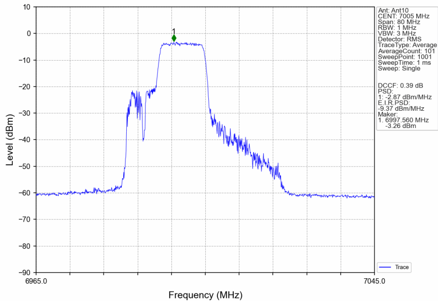
802.11be(EHT40)_MCH_7005MHz_26+106 / Ant10_NTNV
