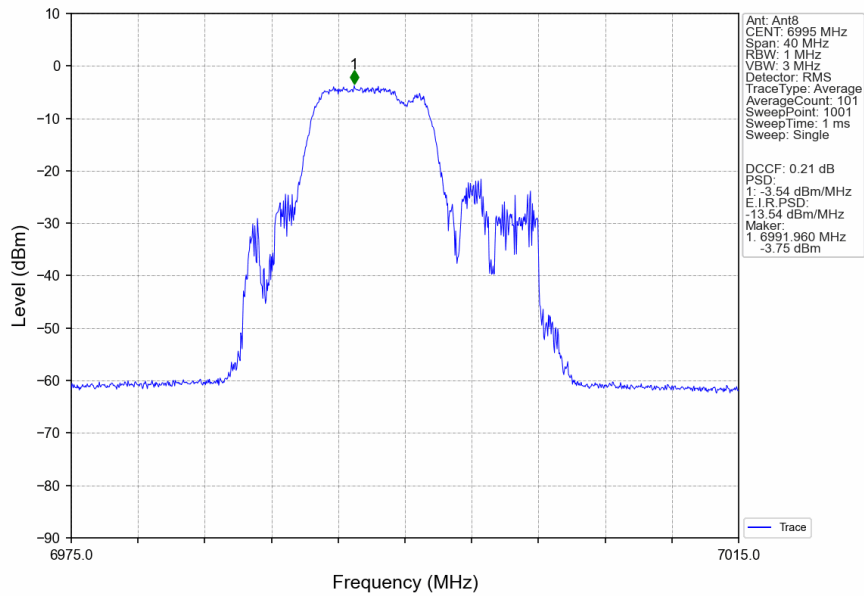
802.11be(EHT20)_MCH_6995MHz_26+52_/_MIMO_NTNV
