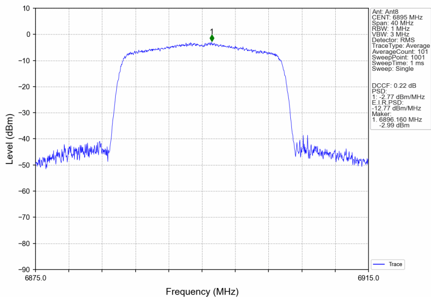
802.11be(EHT20)_LCH_6895MHz_RU242_Left_Ant8_NTNV
