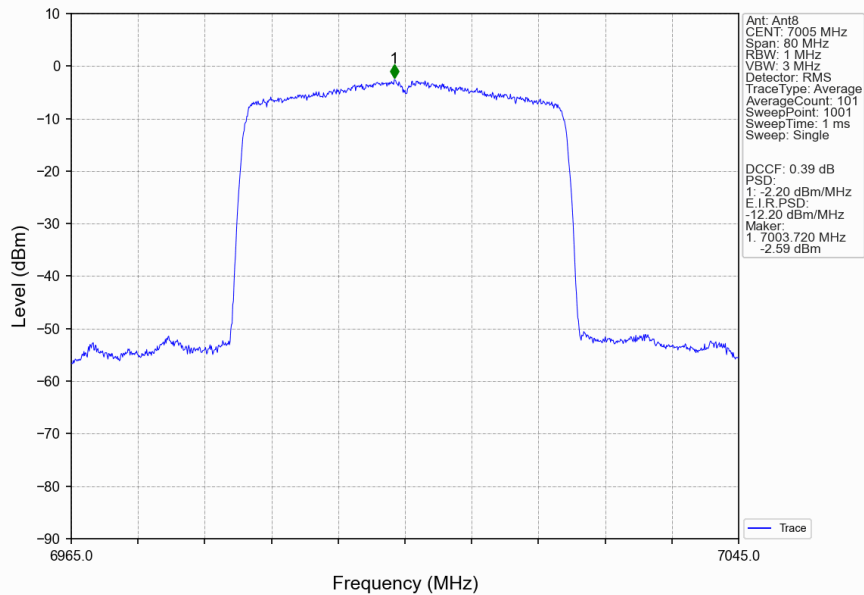
802.11be(EHT40)_MCH_7005MHz_RU484_Left_Ant8_NTNV
