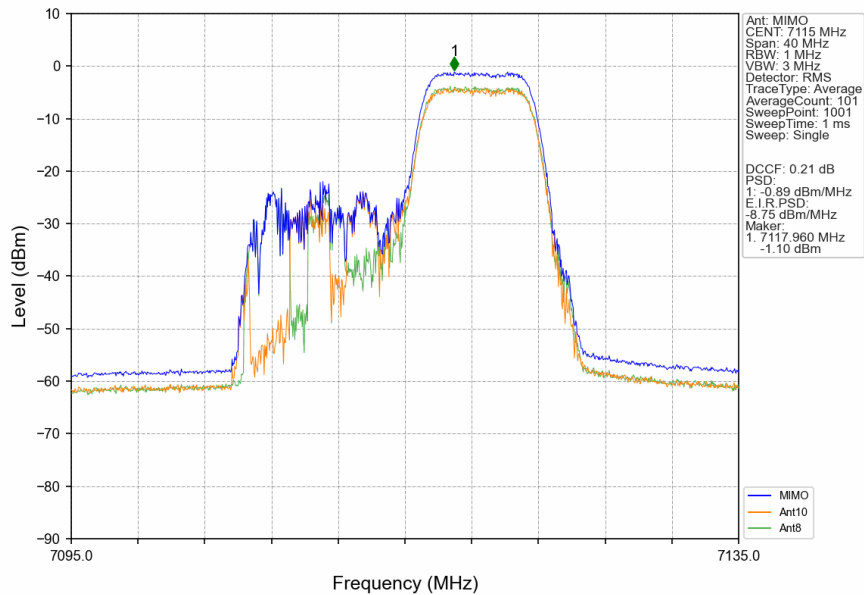
802.11be(EHT20)_HCH_7115MHz_26+52_/_MIMO_NTNV
