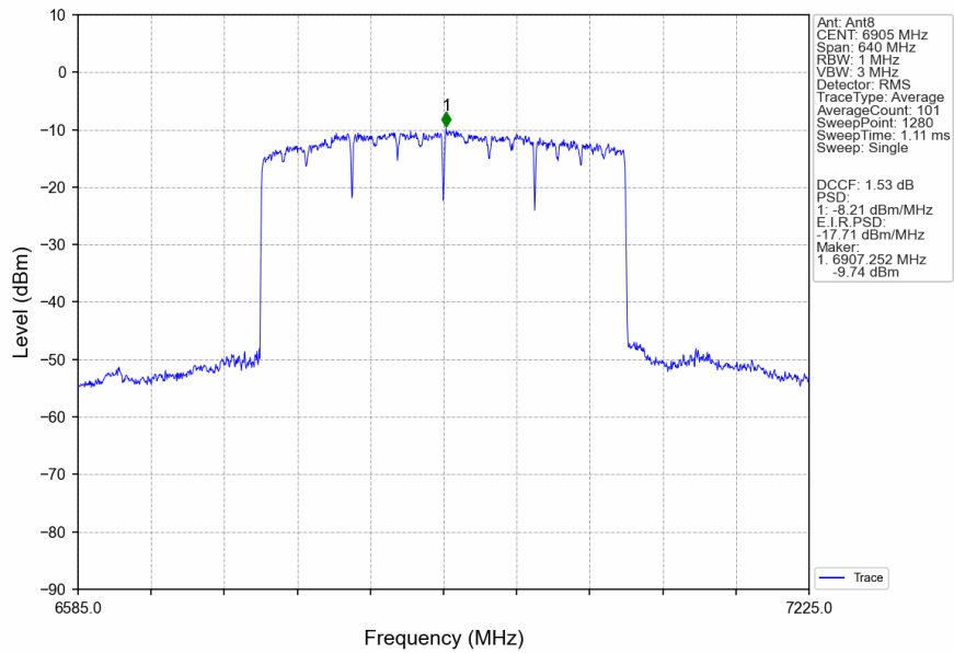
802.11be(EHT320)_HCH_6905MHz_4xRU996_Left_MIMO_NTNV
