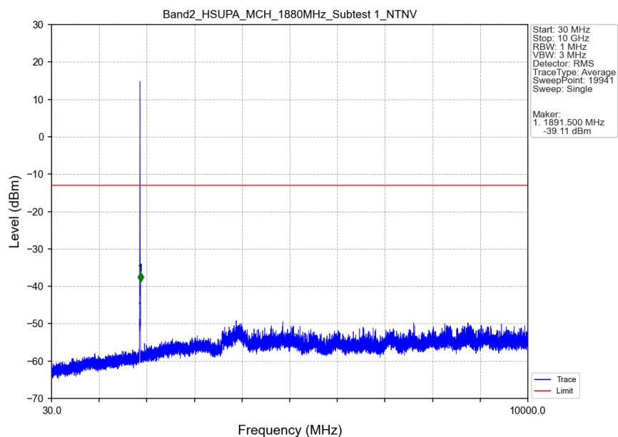
Band2_HSUPA_MCH_1880MHz_Subtest 1_NTNV
