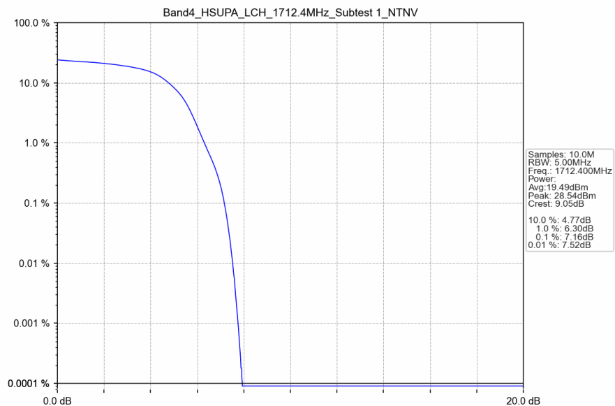
Band4_HSUPA_LCH_1712.4MHz_Subtest 1_NTNV
