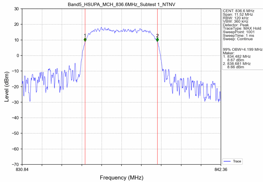
Band5_HSUPA_MCH_836.6MHz_Subtest 1_NTNV
