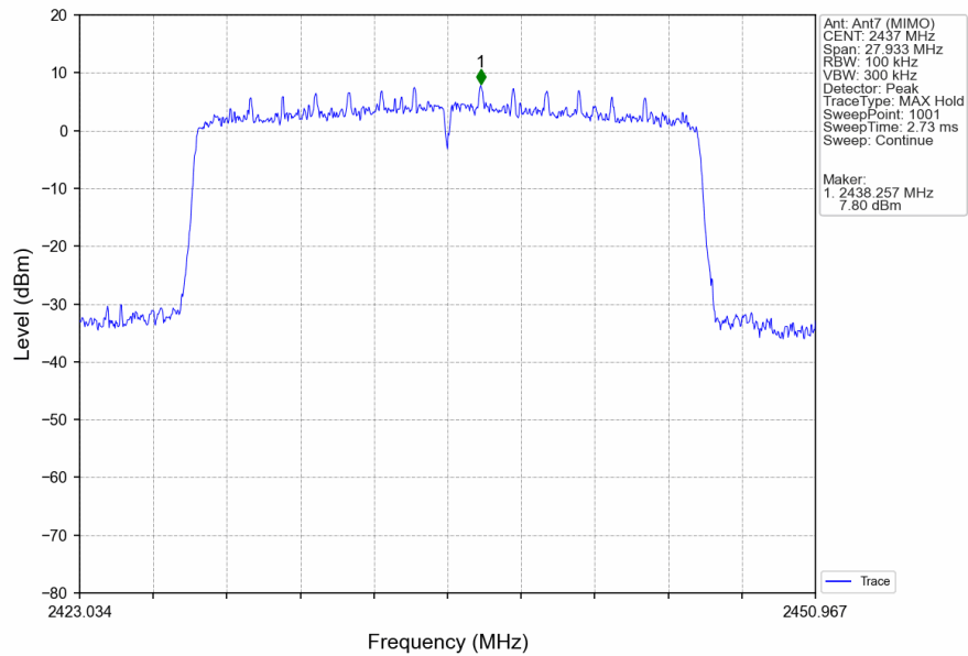
802.11be(EHT20) MCH 2437MHz RU242 Left Ant7 (MIMO) NTN
