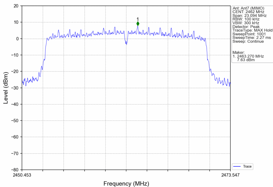
802.11ac(VHT20) HCH 2462MHz Ant7 (MIMO) NTN
