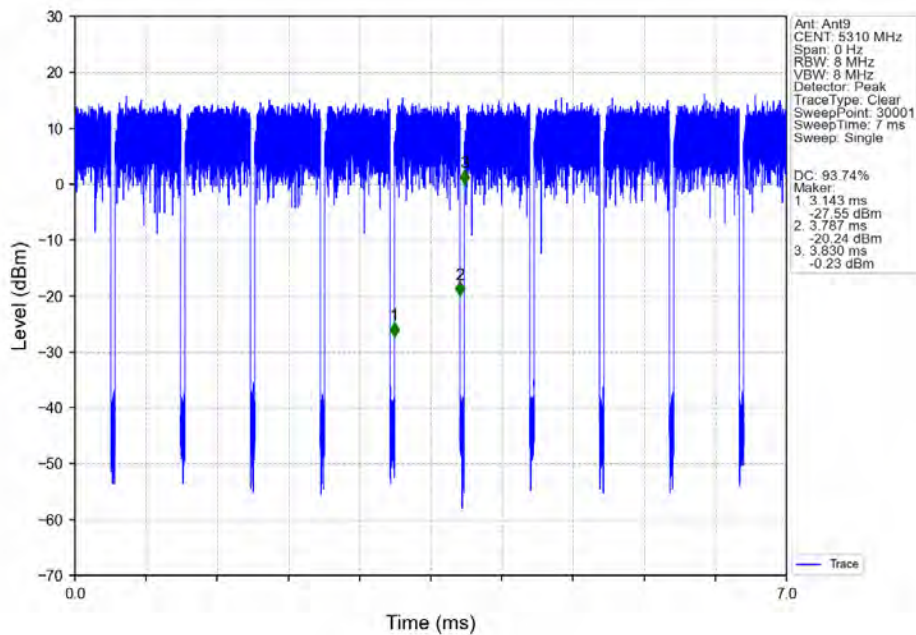
802.11n(HT40)_HCH_5310MHz_Ant9_NTNV
