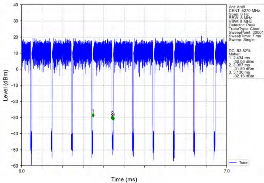
802.11ac(VHT40)_LCH_5270MHz_Ant9_NTNV
