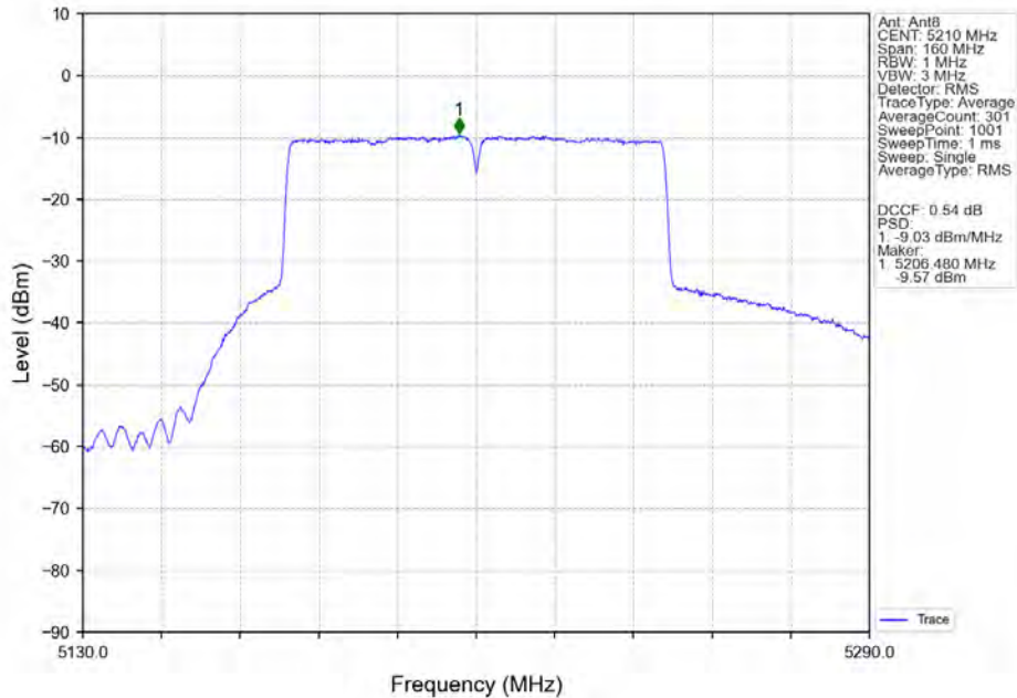
802.11ac(VHT80)_MCH_5210MHz_MIMO_NTNV
