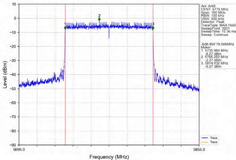
802.11ax(HEW80)_MCH_5775MHz_RU996_Left_Ant9_NTNV
