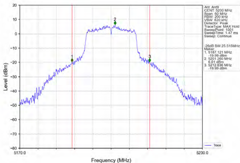
802.11a_MCH_5200MHz_Ant9_NTNV
