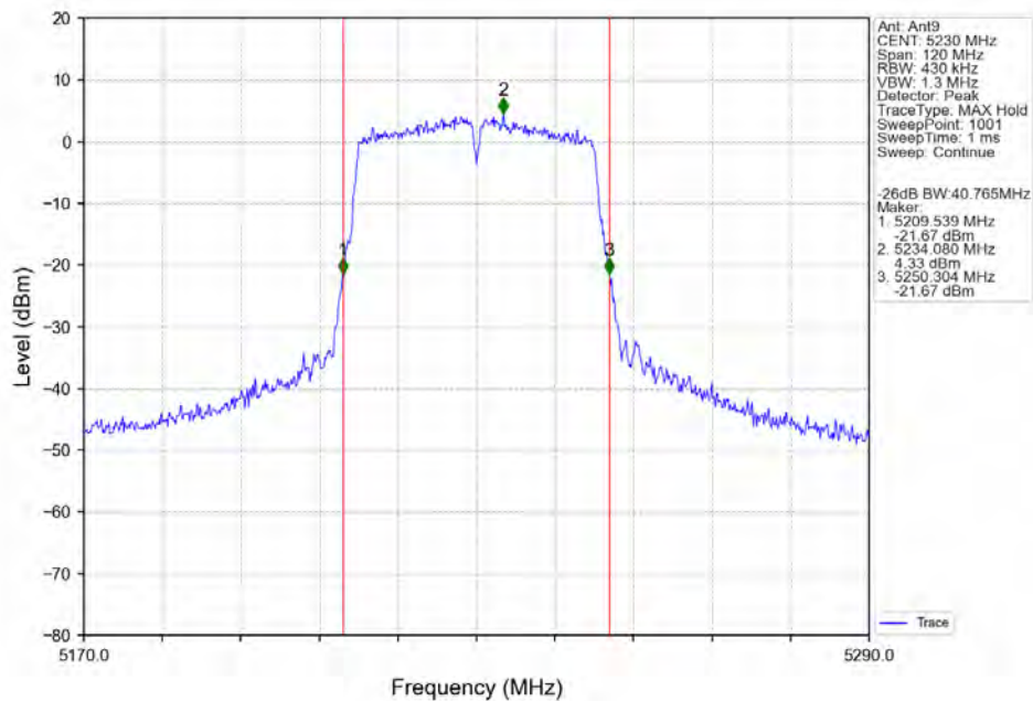
802.11ac(VHT40)_HCH_5230MHz_Ant9_NTNV
