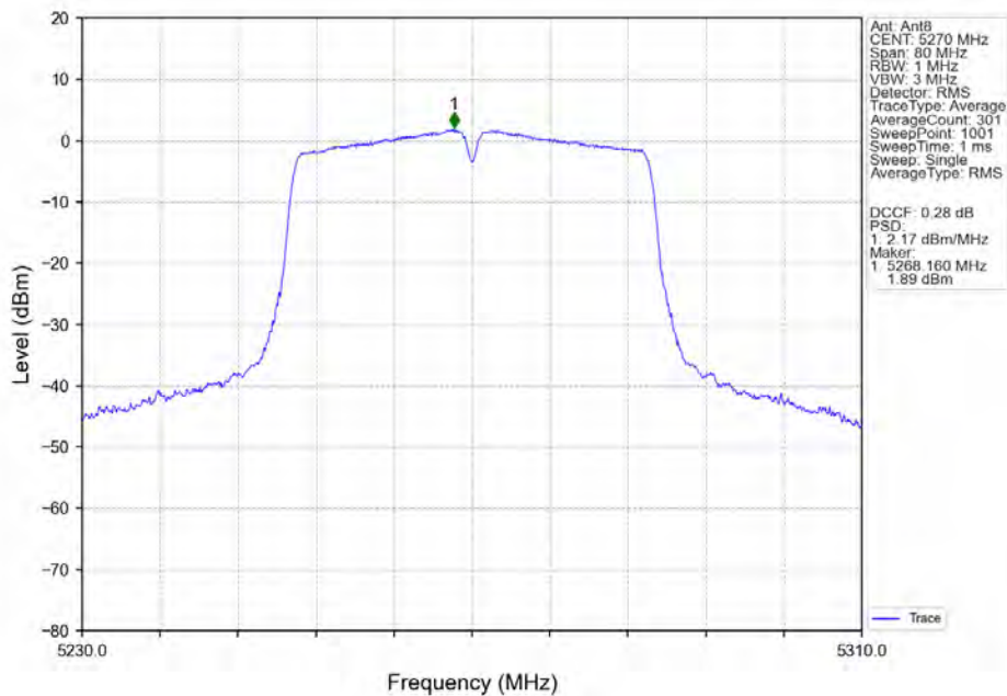
802.11n(HT40)_LCH_5270MHz_Ant8_NTNV
