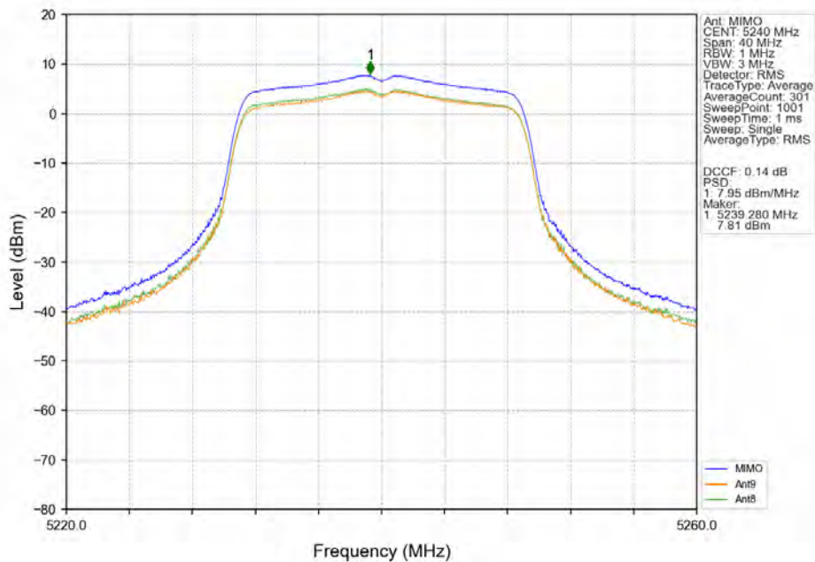
802.11n(HT20)_HCH_5240MHz_MIMO_NTNV
