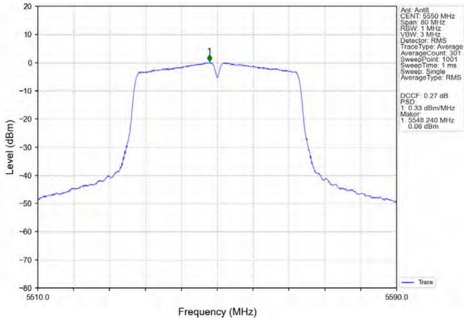
802.11n(HT40)_MCH_5550MHz_MIMO_NTNV
