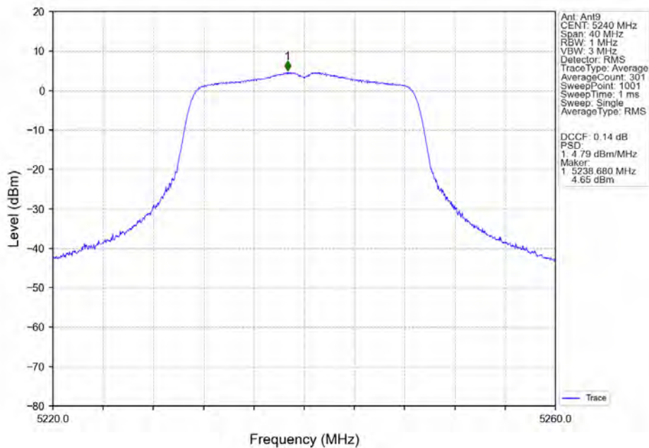
802.11n(HT20)_HCH_5240MHz_Ant9_NTNV
