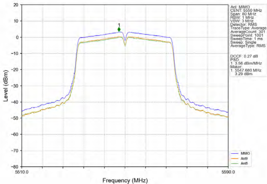
802.11n(HT40)_MCH_5550MHz_MIMO_NTNV
