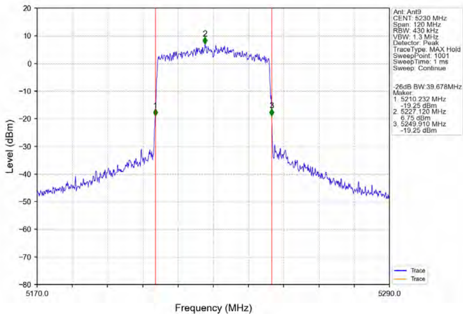
802.11ax(HEW40)_HCH_5230MHz_RU484_Left_Ant9_NTNV
