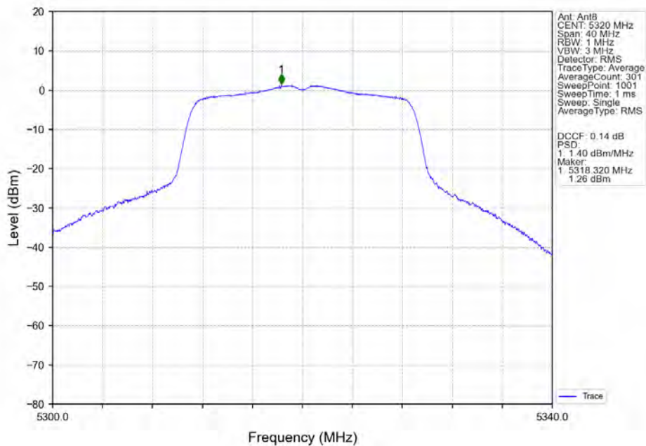
802.11ac(VHT20)_HCH_5320MHz_Ant8_NTNV
