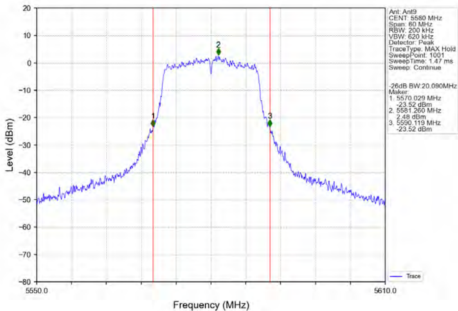
802.11a_MCH_5580MHz_Ant9_NTNV
