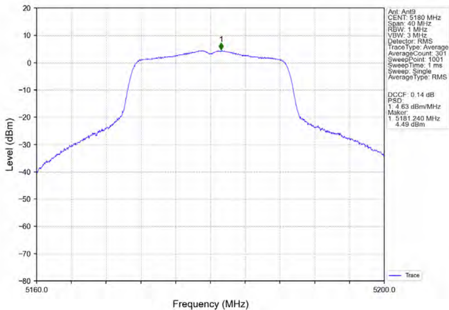
802.11n(HT20)_LCH_5180MHz_Ant9_NTNV
