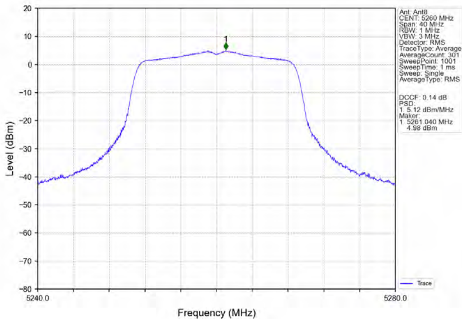
802.11n(HT20)_LCH_5260MHz_Ant8_NTNV
