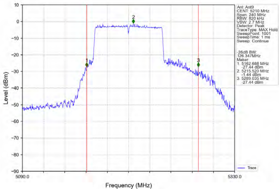
802.11ac(VHT80)_MCH_5210MHz_Ant9_NTNV
