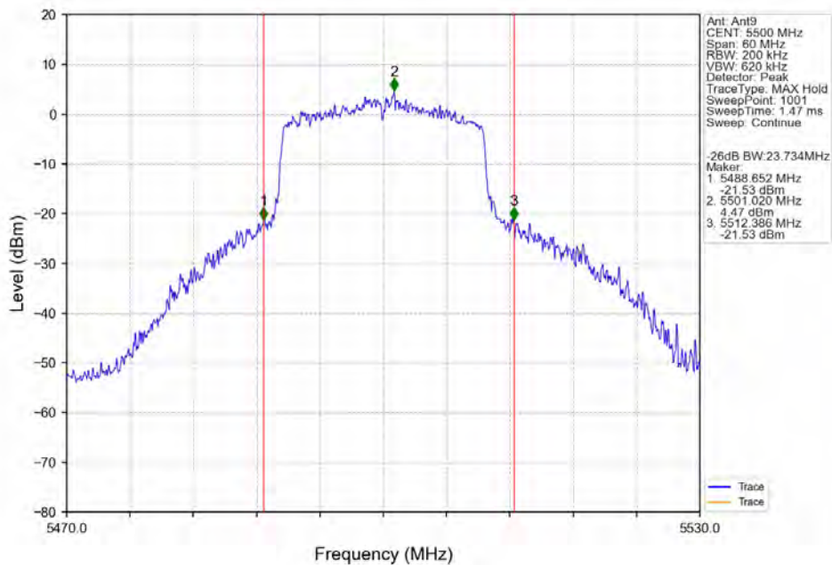
802.11ax(HEW20)_LCH_5500MHz_RU242_Left_Ant9_NTNV
