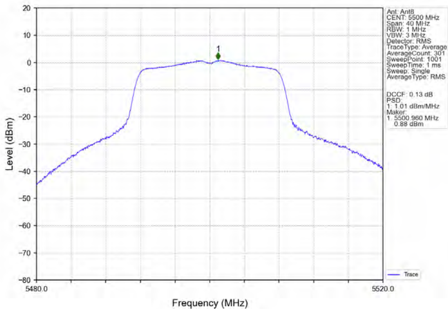
802.11a_LCH_5500MHz_Ant8_NTNV
