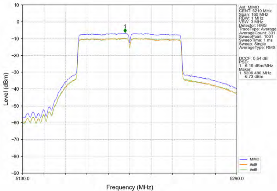
802.11ac(VHT80)_MCH_5210MHz_MIMO_NTNV
