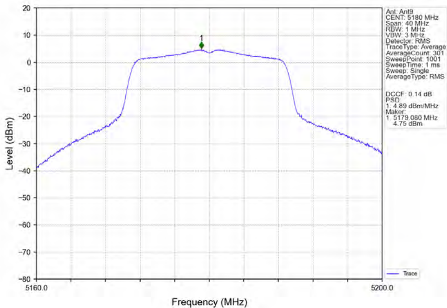
802.11ac(VHT20)_LCH_5180MHz_Ant9_NTNV
