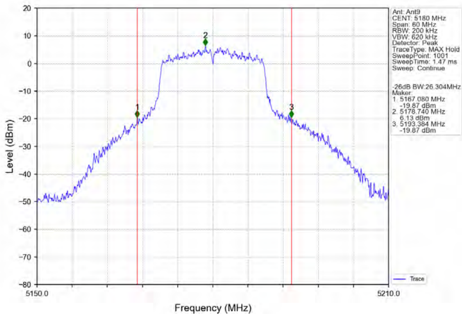
802.11n(HT20)_LCH_5180MHz_Ant9_NTNV
