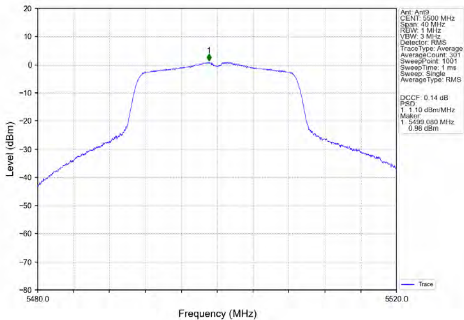
802.11n(HT20)_LCH_5500MHz_Ant9_NTNV
