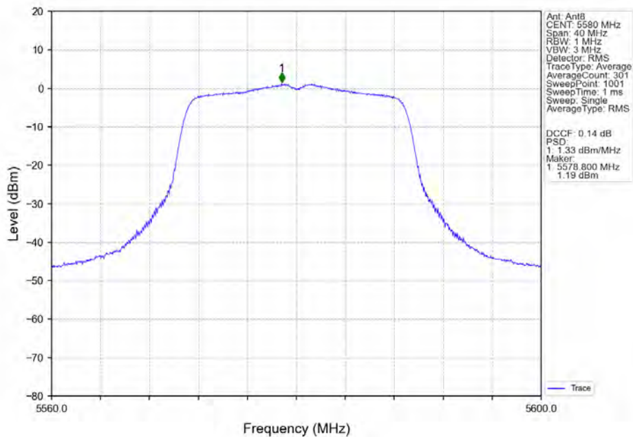
802.11n(HT20)_MCH_5580MHz_Ant8_NTNV
