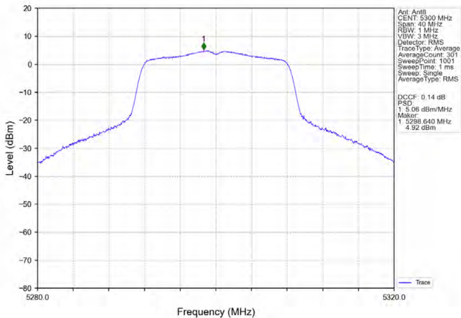
802.11a_MCH_5300MHz_Ant8_NTNV
