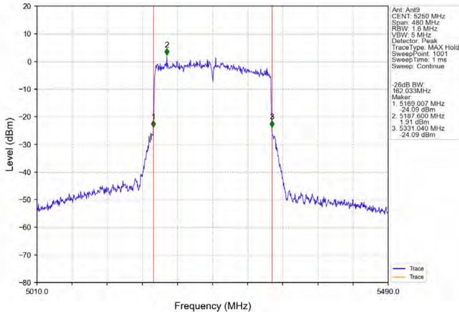
802.11ax(HEW160)_MCH_5250MHz_2xRU996_Left_Ant9_NTNV
