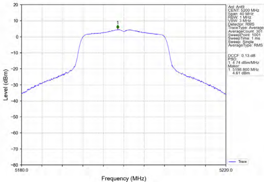
802.11a_MCH_5200MHz_Ant9_NTNV
