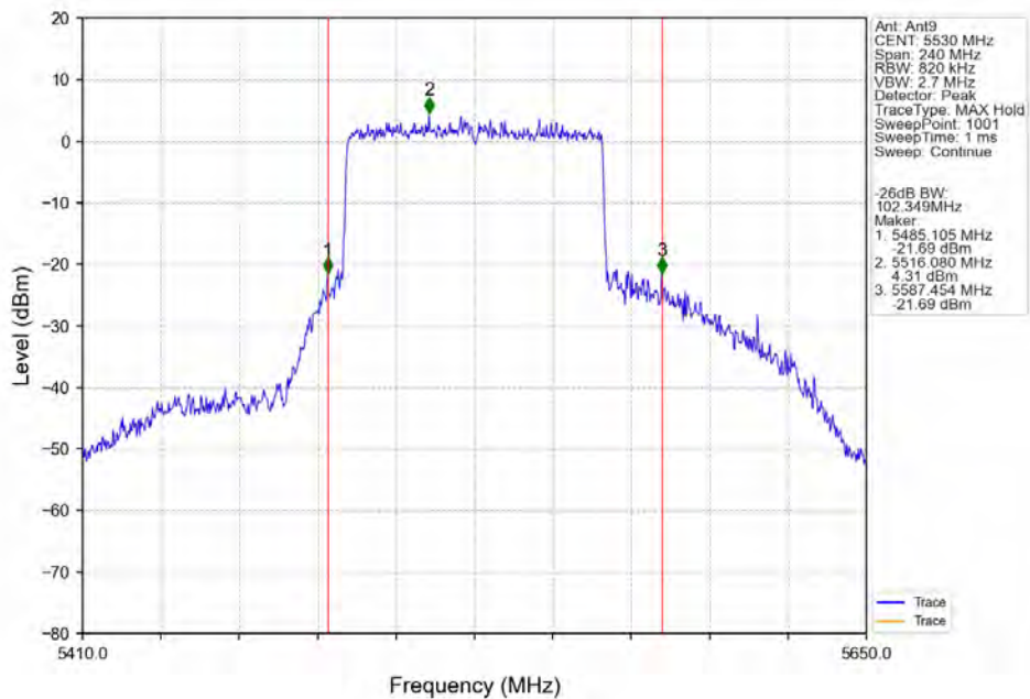
802.11ax(HEW80)_LCH_5530MHz_RU996_Left_Ant9_NTNV
