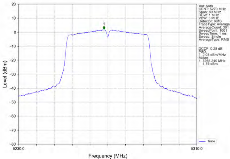
802.11ac(VHT40)_LCH_5270MHz_Ant8_NTNV
