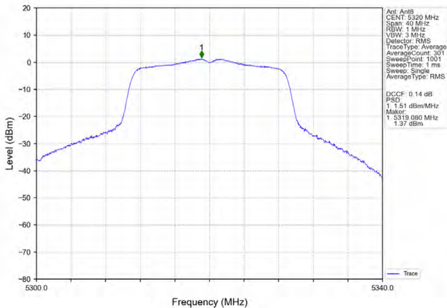
802.11n(HT20)_HCH_5320MHz_Ant8_NTNV
