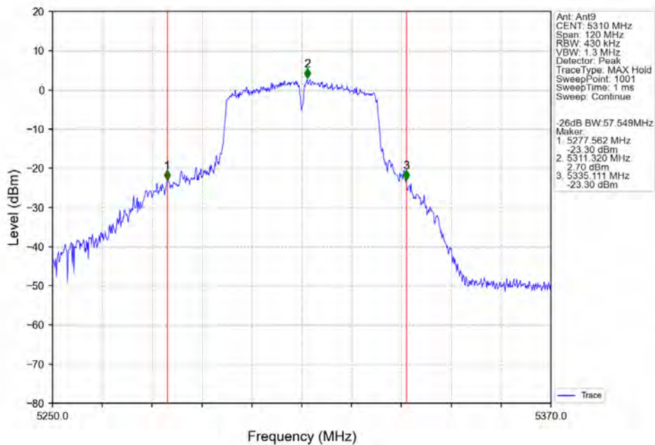
802.11n(HT40)_HCH_5310MHz_Ant9_NTNV
