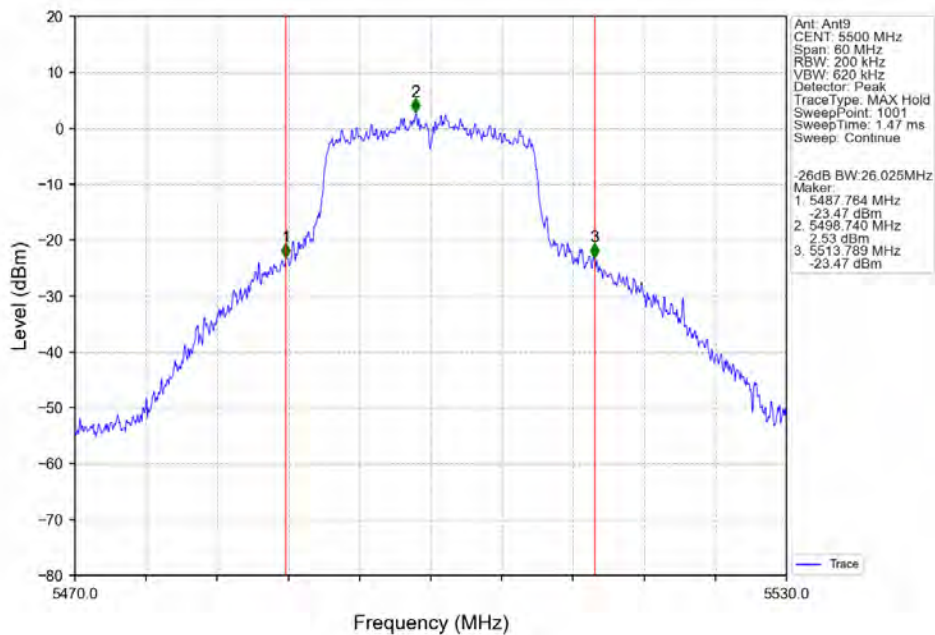
802.11n(HT20)_LCH_5500MHz_Ant9_NTNV
