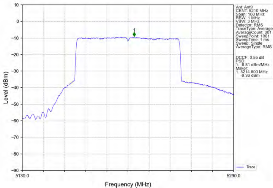
802.11ax(HEW80)_MCH_5210MHz_RU996_Left_Ant9_NTNV
