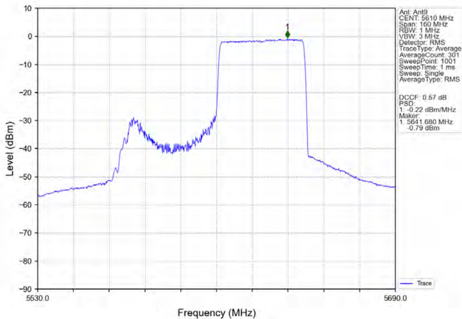
802.11ax(HEW80)_HCH_5610MHz_RU484_Right_Ant9_NTNV
