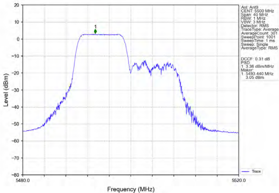
802.11ax(HEW20)_LCH_5500MHz_RU106_Left_Ant9_NTNV
