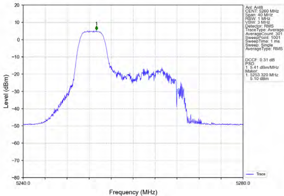
802.11ax(HEW20)_LCH_5260MHz_RU52_Left_Ant8_NTNV
