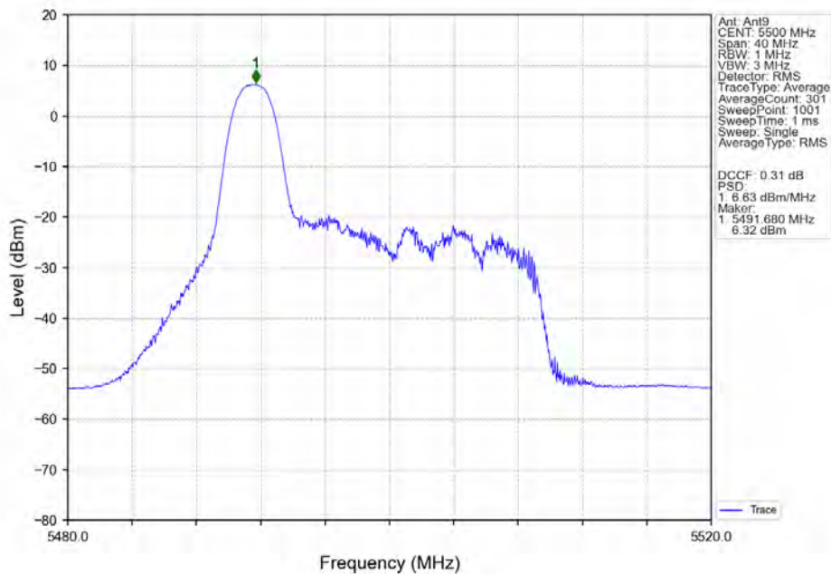
802.11ax(HEW20)_LCH_5500MHz_RU26_Left_Ant9_NTNV
