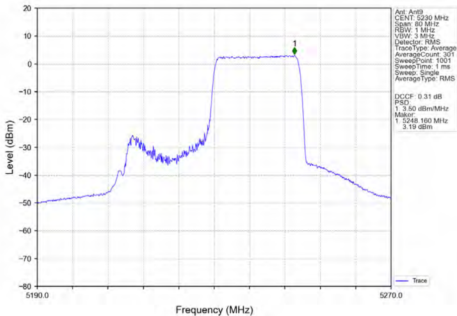
802.11ax(HEW40)_HCH_5230MHz_RU242_Right_Ant9_NTNV
