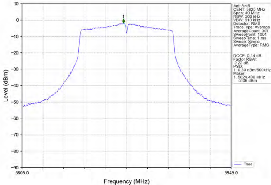
802.11n(HT20)_HCH_5825MHz_MIMO_NTNV
