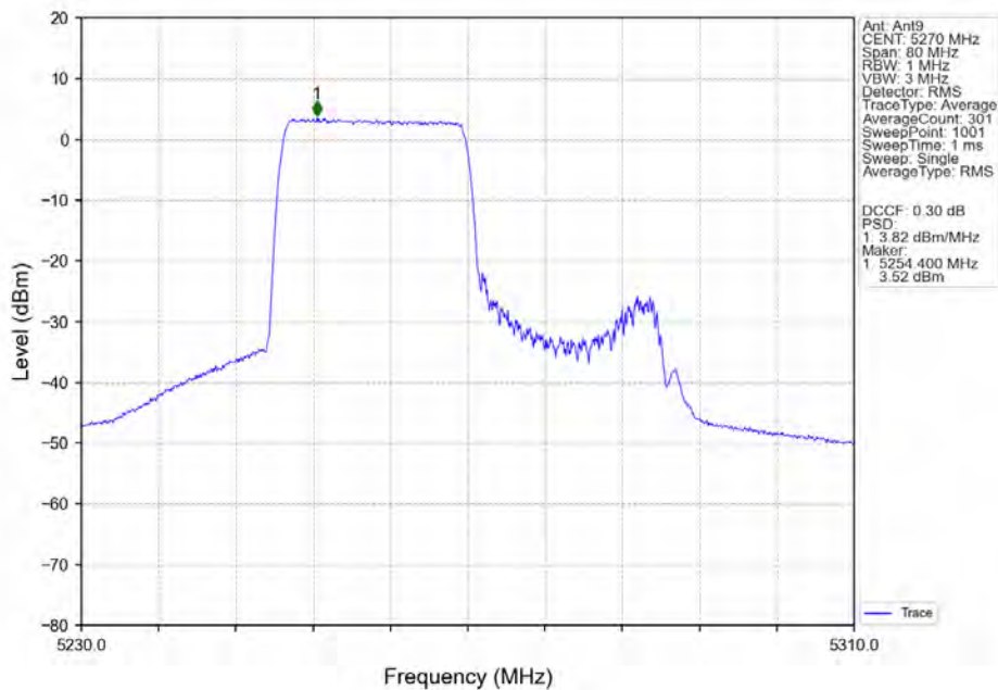
802.11ax(HEW40)_LCH_5270MHz_RU242_Left_Ant9_NTNV
