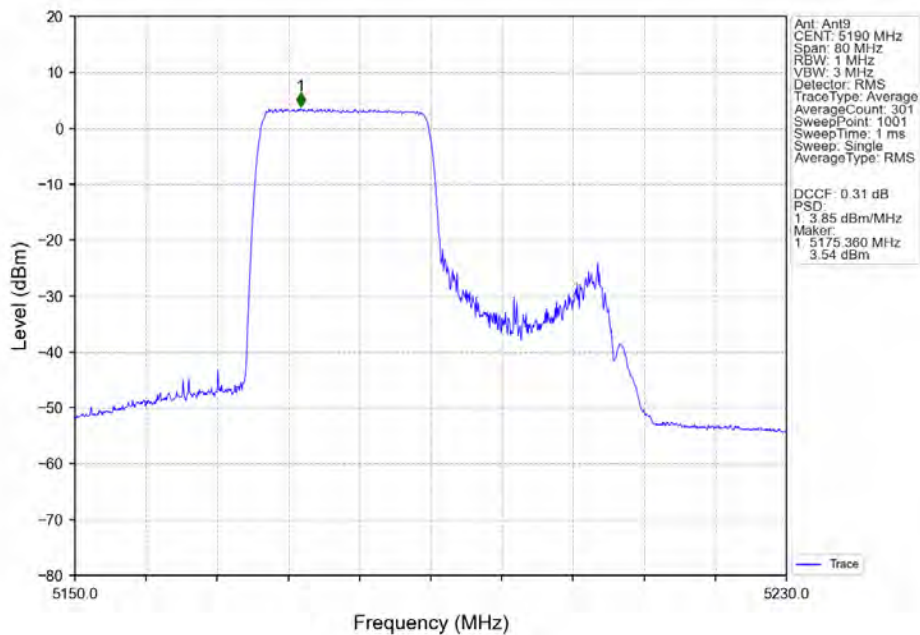
802.11ax(HEW40)_LCH_5190MHz_RU242_Left_Ant9_NTNV
