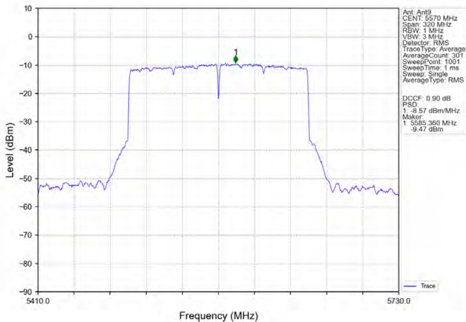
802.11ax(HEW160)_MCH_5570MHz_2xRU996_Left_Ant9_NTNV
