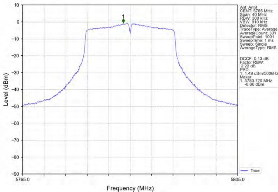
802.11a_MCH_5785MHz_Ant9_NTNV
