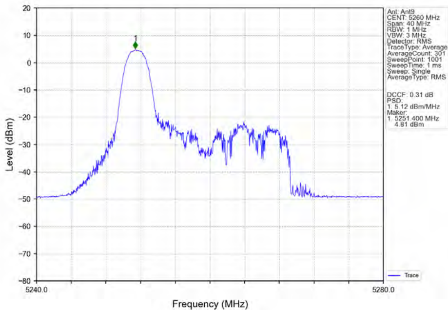
802.11ax(HEW20)_LCH_5260MHz_RU26_Left_Ant9_NTNV
