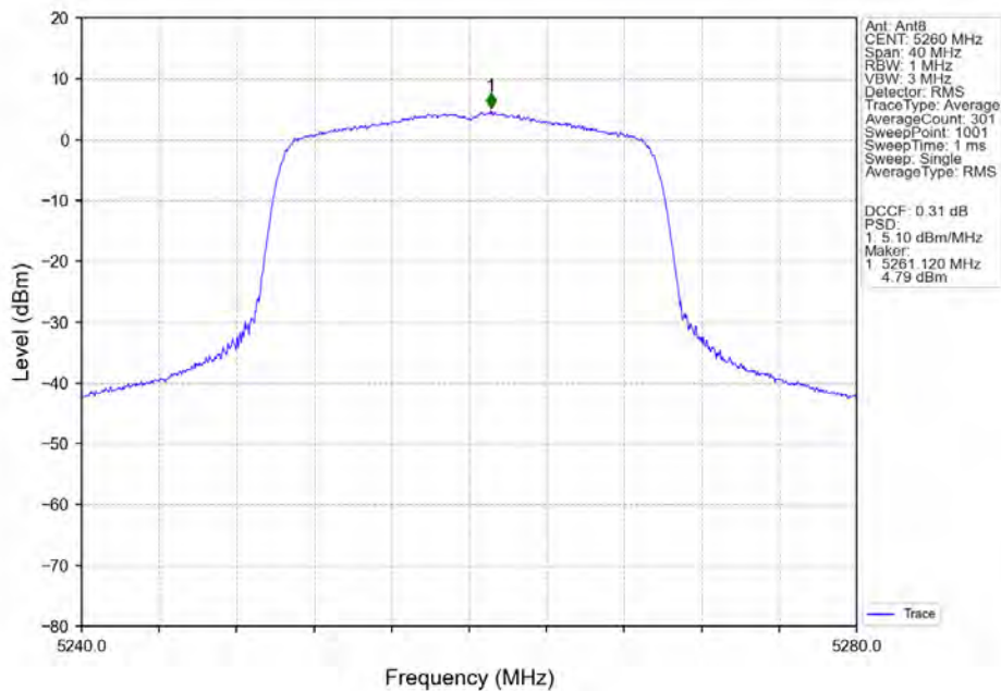
802.11ax(HEW20)_LCH_5260MHz_RU242_Left_Ant8_NTNV
