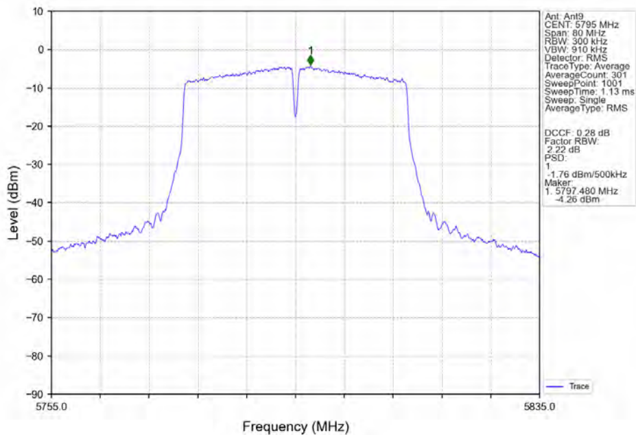
802.11n(HT40)_HCH_5795MHz_Ant9_NTNV
