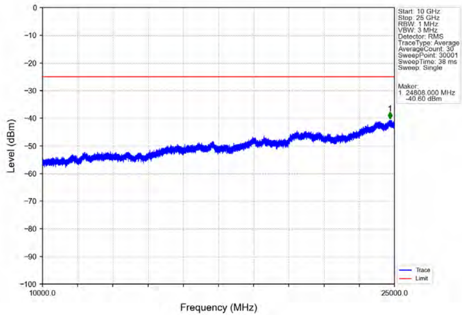
Band7_20MHz_64QAM_MCH_2535MHz_RB_1_0_NTV
