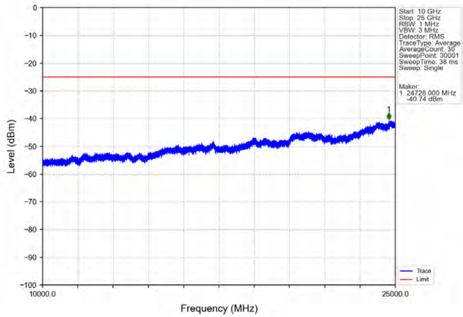
Band7 10MHz 64QAM MCH 2535MHz RB 1 0 NTNV
