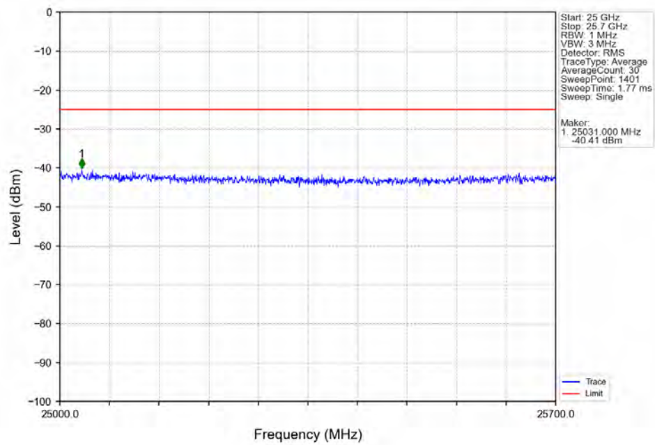
Band7 20MHz 64QAM LCH 2510MHz RB 1 0 NTNV
