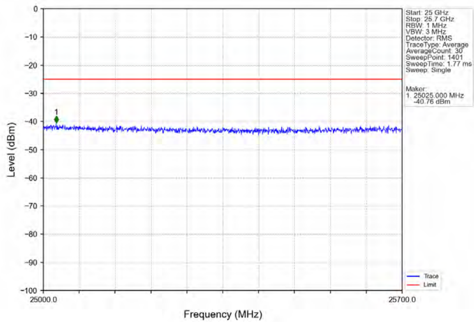
Band7_20MHz_64QAM_MCH_2535MHz_RB_1_0_NTV
