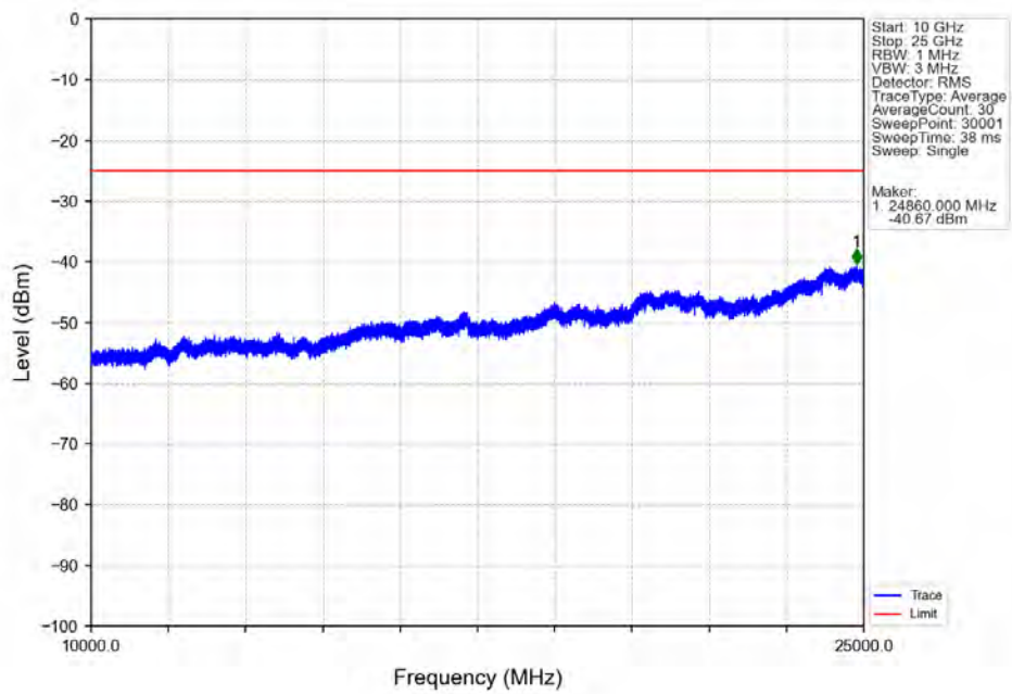
Band7 10MHz 16QAM MCH 2535MHz RB 1 0 NTNV
