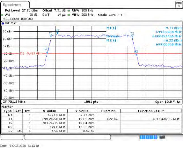
1-N12-PC3-15-5-L-3-DFT-16QAM-Outer_Full-25@0-Ant0-4.505-4.950-≤5-PASS
