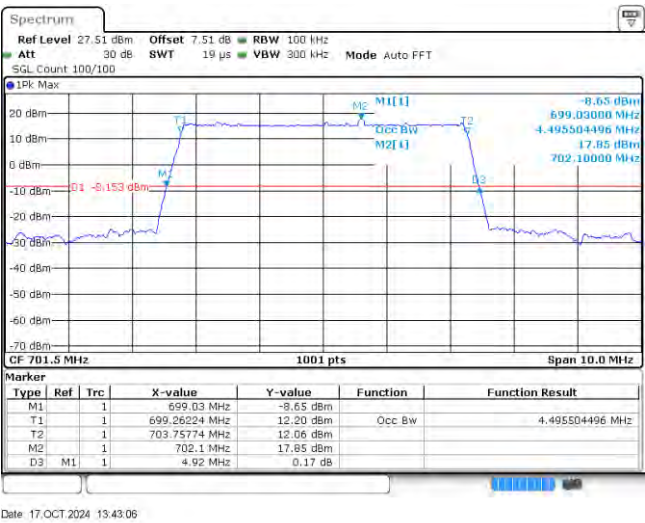
1-N12-PC3-15-5-L-1-DFT-QPSK-Outer_Full-25@0-Ant0-4.496-4.920-≤5-PASS
