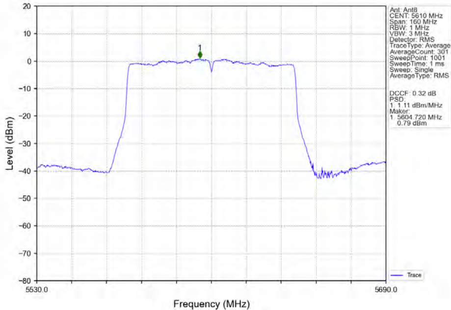
802.11ac(VHT80)_HCH_5610MHz_Ant8_NTNV
