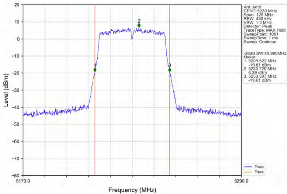
802.11ac(VHT40) HCH 5230MHz_Ant8_NTNV
