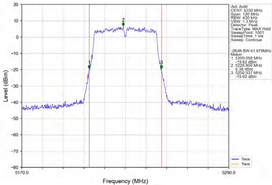
802.11n(HT40) HCH 5230MHz Ant8 NTN
