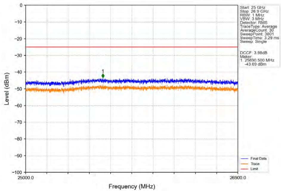
Band41_15MHz_QPSK_MCH_2593MHz_RB_1_0_NTNV
