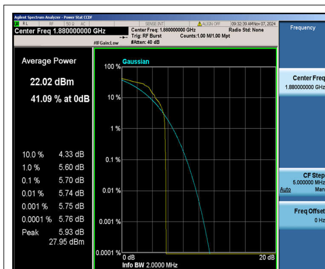
EGPRS1900-661-2
