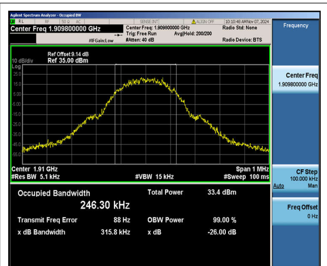
GSM1900-810-0-0.3158
