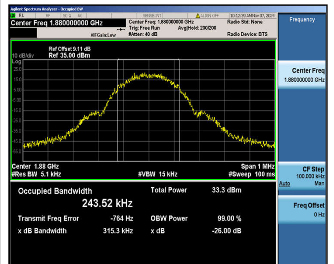
GPRS1900-661-0-0.3153
