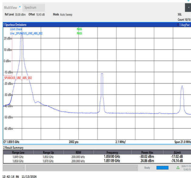
Band2_20MHz_QPSK_18700_1RB#0
