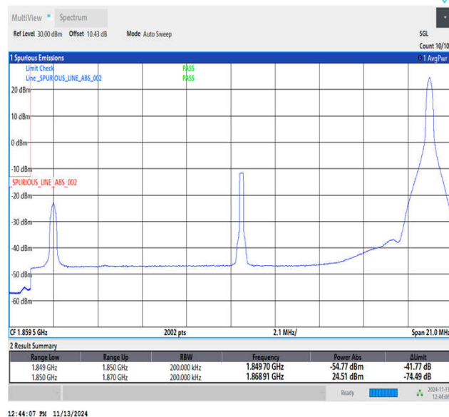
Band2_20MHz_QPSK_18700_1RB#99
