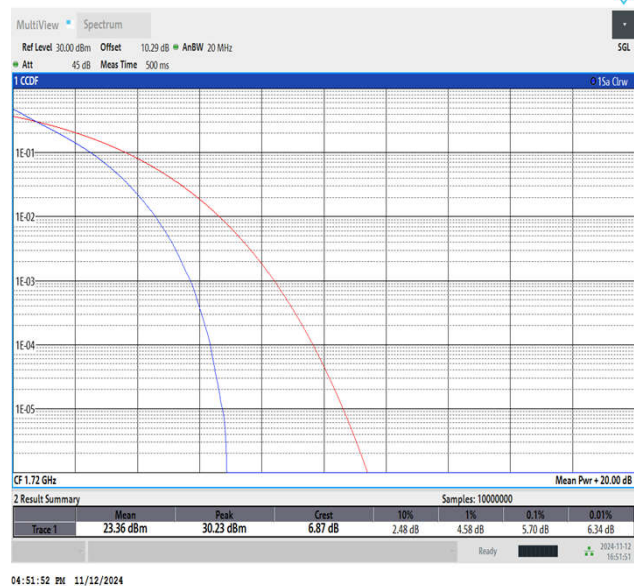
Band4-20MHz-QPSK-20050-100RB#0-PASS
