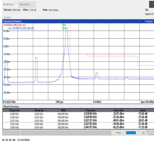
Band38_20MHz_QPSK_38150_1RB#99
