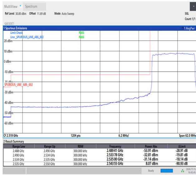
Band41_15MHz_QPSK_40115_75RB#0
