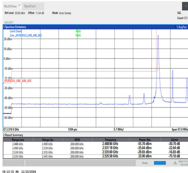
Band41_10MHz_QPSK_40090_1RB#0
