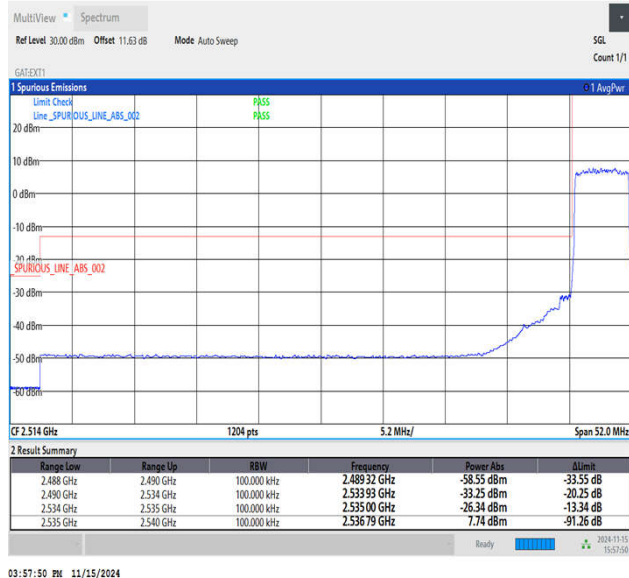
Band41_5MHz_QPSK_40065_25RB#0
