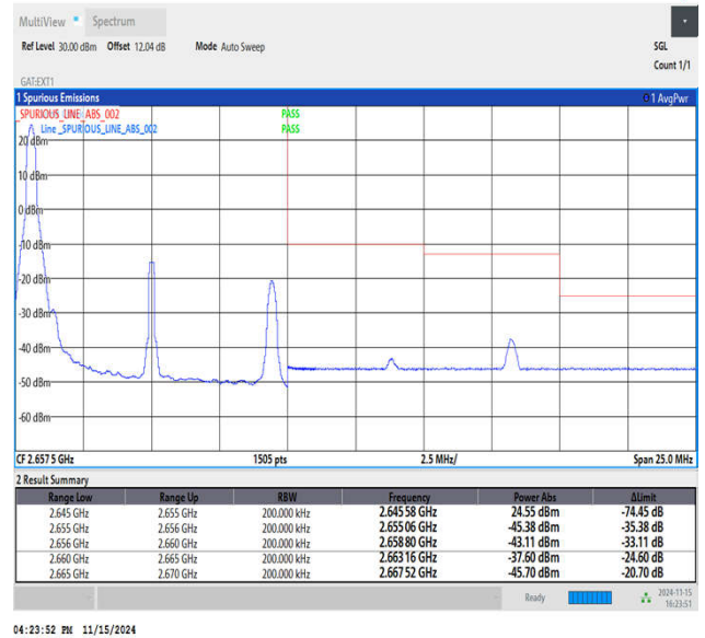
Band41_10MHz_QPSK_41190_1RB#0
