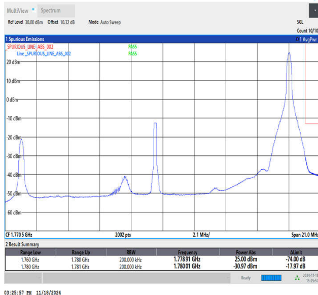
Band66_20MHz_QPSK_132572_1RB#99
