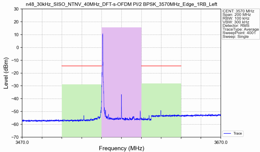
n48_30kHz_SISO_NTNV_40MHz_DFT-s-OFDM PI/2 BPSK_3570MHz_Edge_1RB_Left_Ant6
