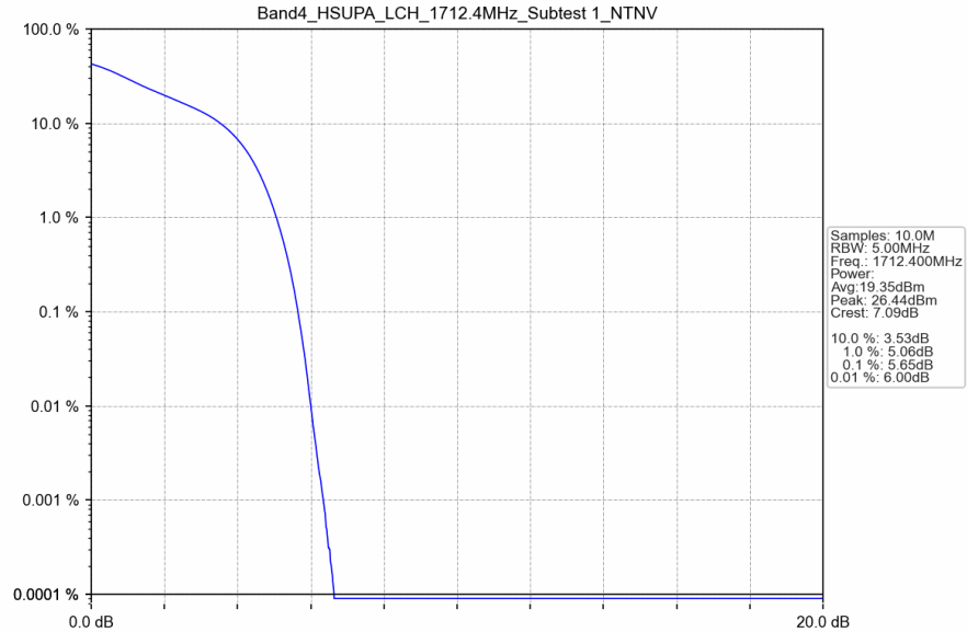
Band4_HSUPA_LCH_1712.4MHz_Subtest 1_NTNV
