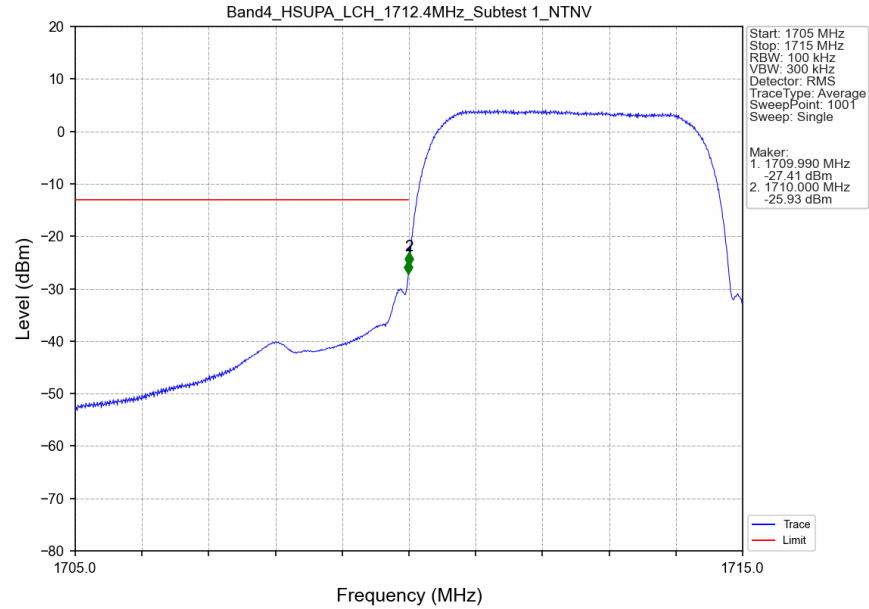
Band4_HSUPA_LCH_1712.4MHz_Subtest 1_NTNV
