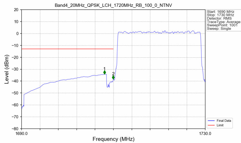
Band4 20MHz QPSK LCH 1720MHz RB 100 0 NTN
