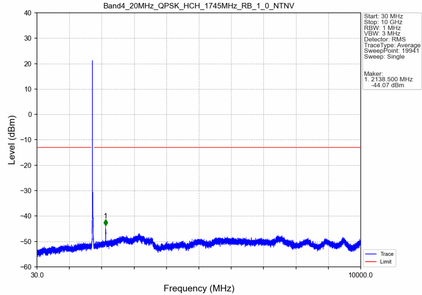
Band4_20MHz_QPSK_HCH_1745MHz_RB_1_0_NTNV
