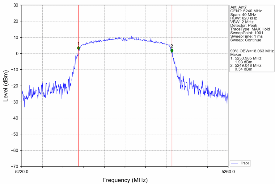
802.11ac(VHT20) HCH 5240MHz Ant7 NTN
