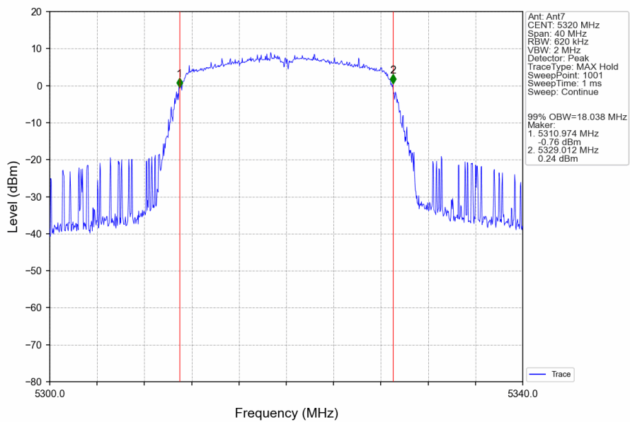
802.11n(HT20) HCH 5320MHz Ant7 NTN
