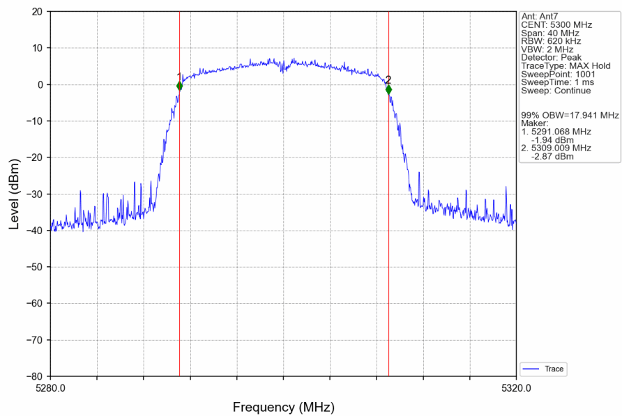
802.11ac(VHT20) MCH 5300MHz Ant7 NTN
