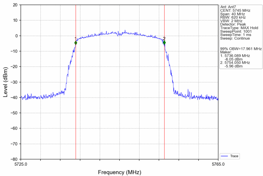
802.11n(HT20) LCH 5745MHz Ant7 NTN
