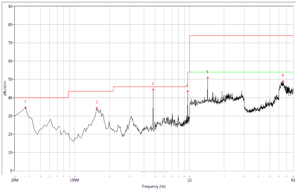
(Plot A: 30MHz – 8GHz, Test Antenna Vertical)
