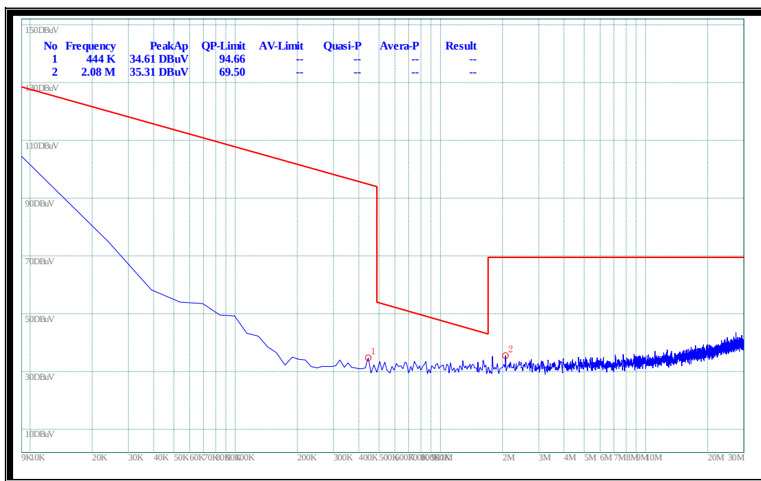
(Plot H.1: 9kHz to 30MHz)
