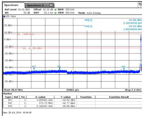
Figure 7.5.1.2-7: 802.11b - 2462MHz - 30MHz - 2.5GHz
