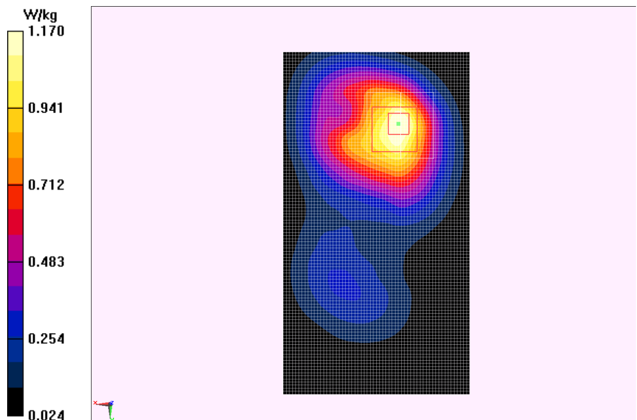
Fig.8 WCDMA1900 CH9262
