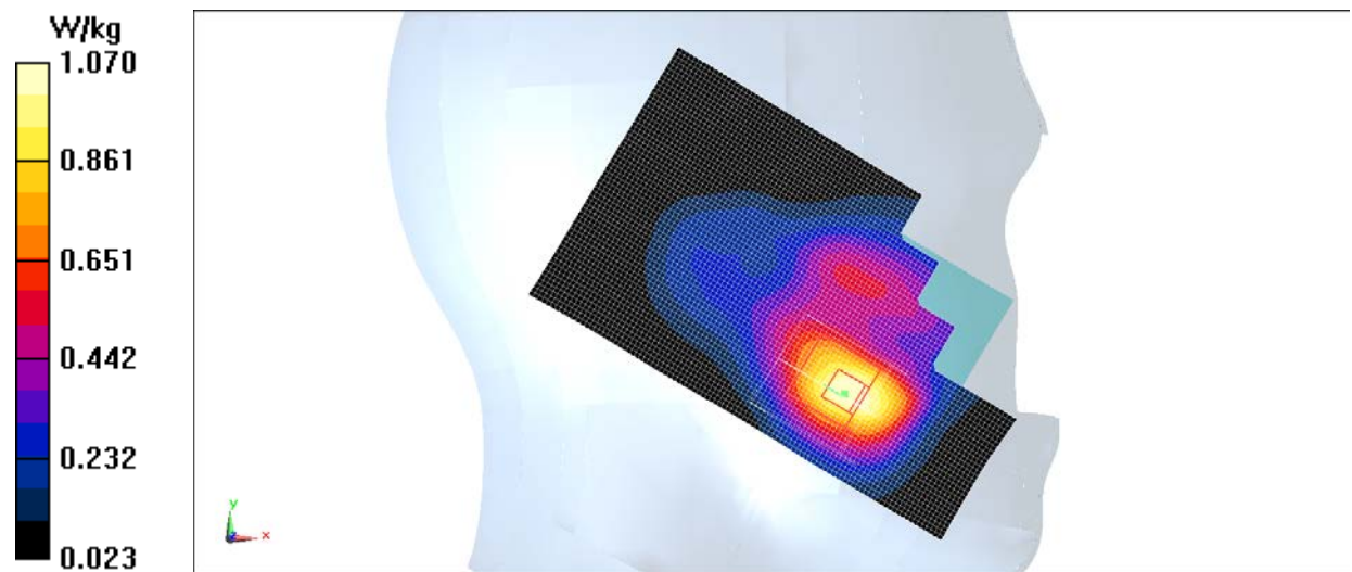
Fig.7 WCDMA1700
