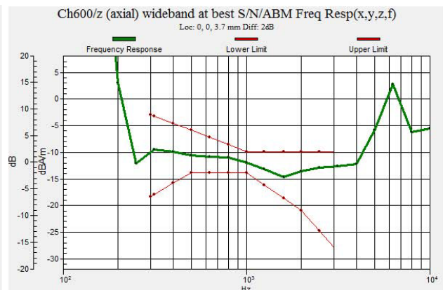
Fig 7.2 CDMA2000 BC1 Ch600
