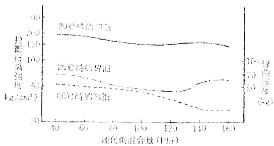
圖 II 2.1 硬化劑混合量和粘附力強度 (在20°C七天的硬化) 試驗片：軟銅板 (25×100×1.6mm) (Over-lap)12.5mm
