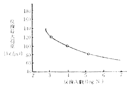
圖 II 2.6 老化特性
