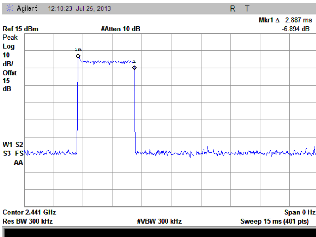
(Plot B: 2DH5 @ \pi/4 -DQPSK)
