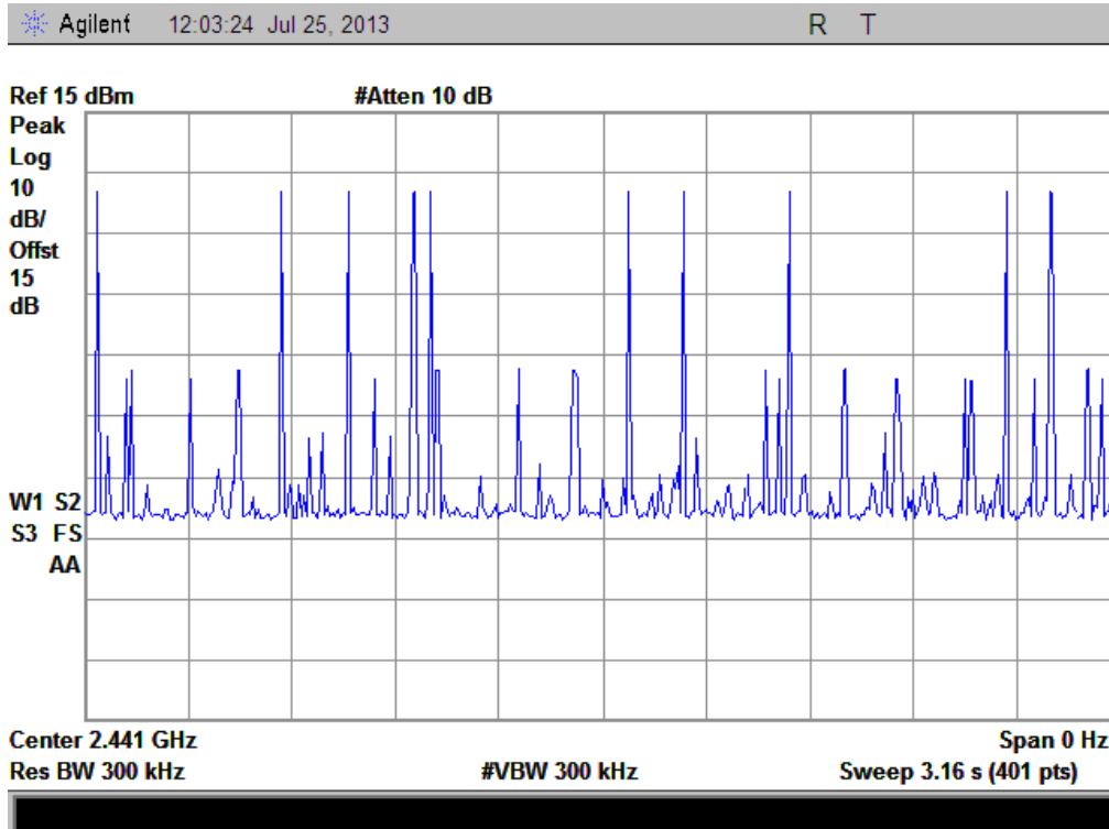
(Plot A: 1DH5 @ GFSK)
