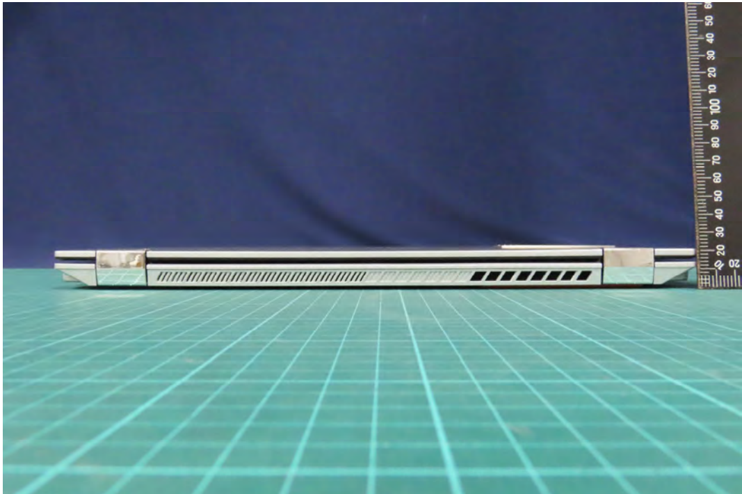
(5) EUT Photo
