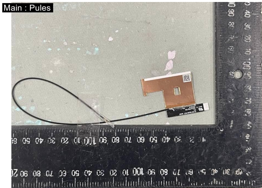
EUT Photo (36)
