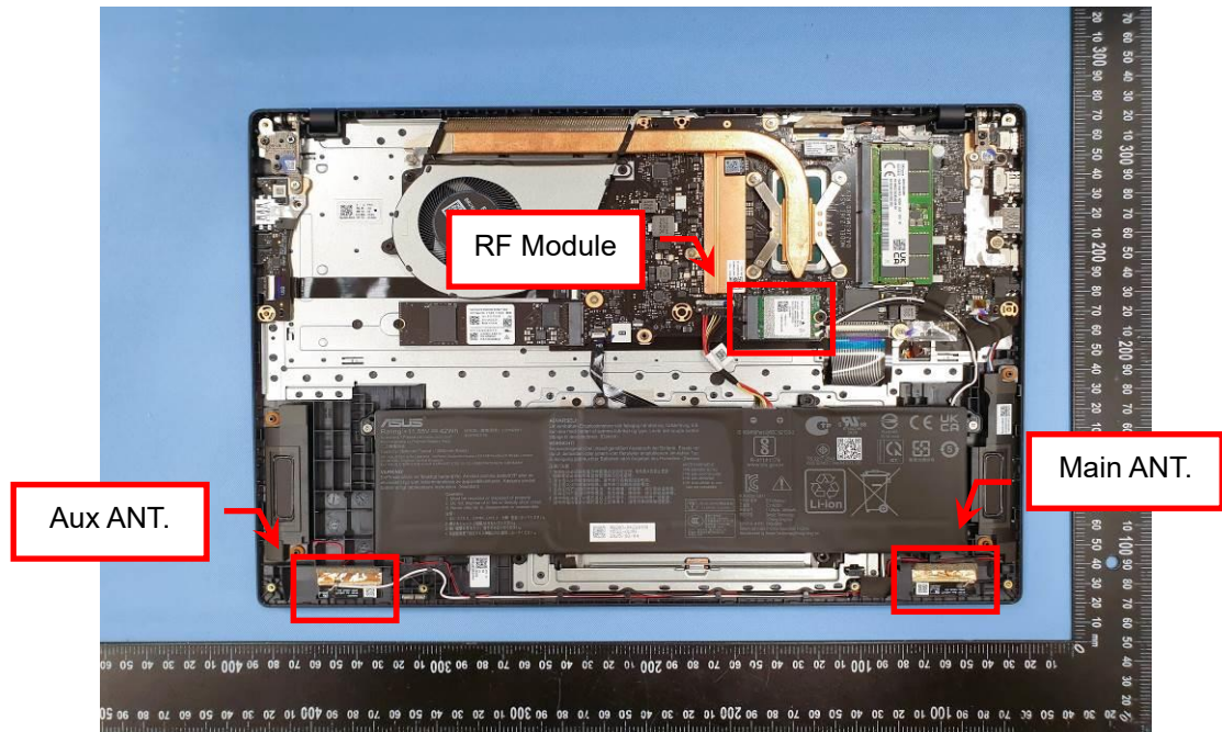
EUT Photo (2)
