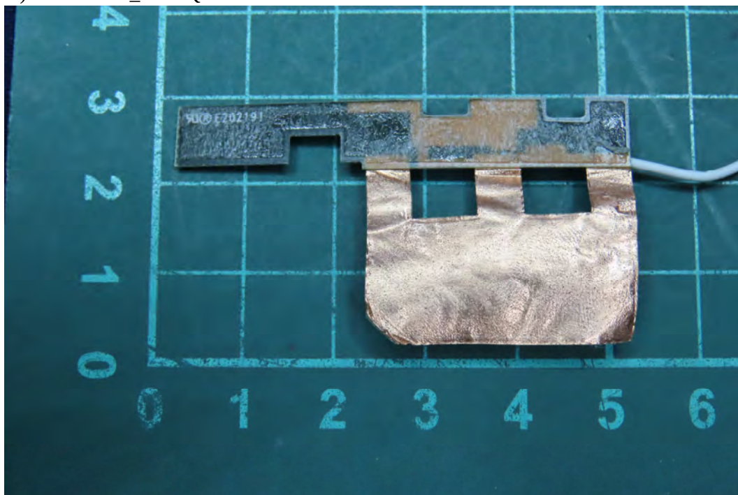
(27) EUT Photo_INPAQ Aux Antenna
