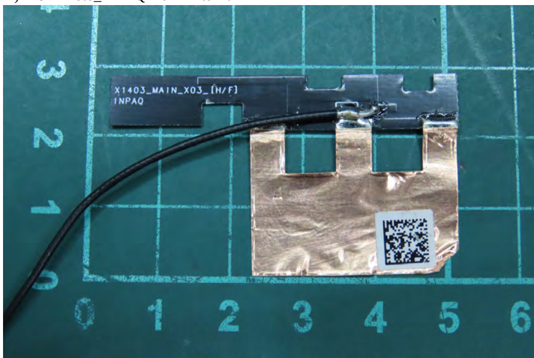
(24) EUT Photo_INPAQ Main Antenna
