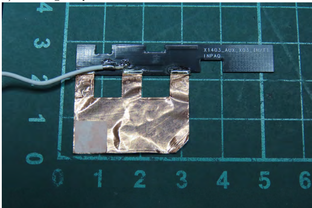
(26) EUT Photo_INPAQ Aux Antenna
