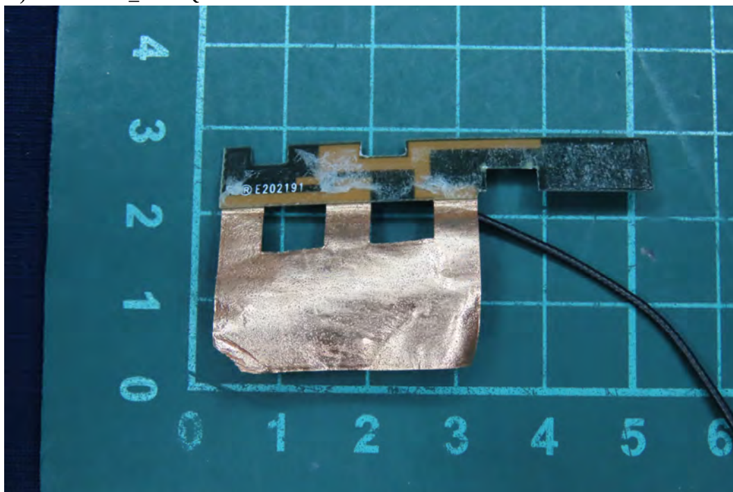
(25) EUT Photo_INPAQ Main Antenna
