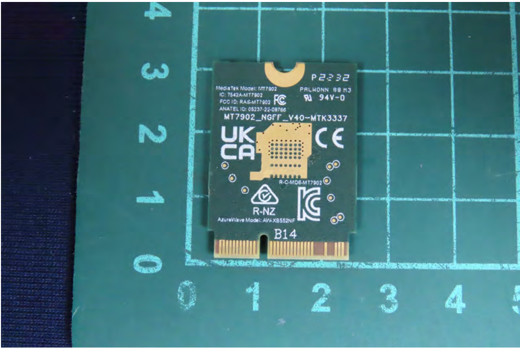
(6) EUT Photo_MT7902
