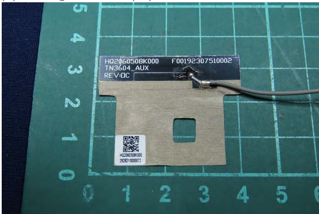
(28) EUT Photo _Antenna: Innowave (Aux)
