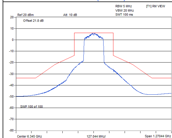
802.11ax (HE160) : CH 79
