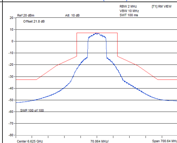
802.11ax (HE80) : CH 135
