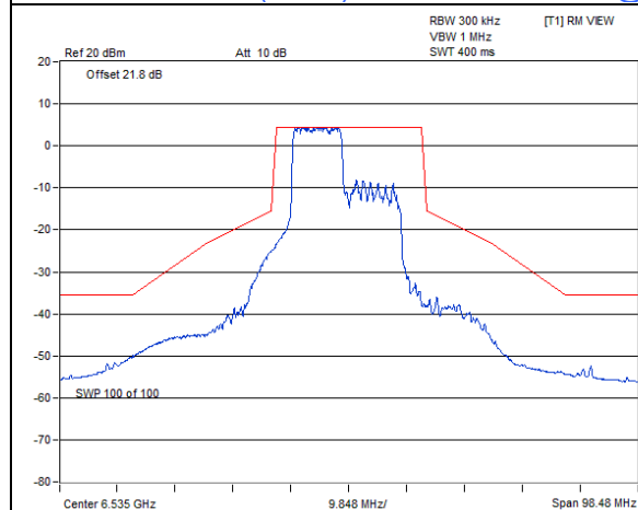
802.11ax (HE20) 106-tone RU : CH 117@53
