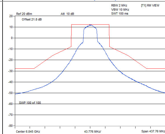
802.11ax (HE40) : CH 179
