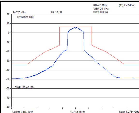
802.11ax (HE160) : CH 47
