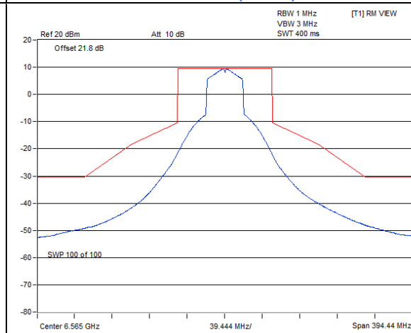
802.11ax (HE40) : CH 123
