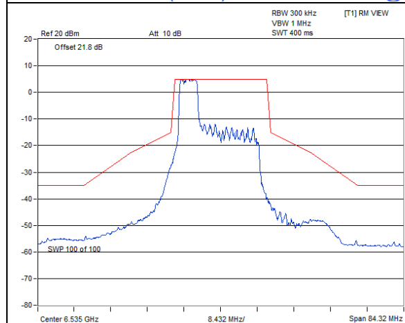
802.11ax (HE20) 52-tone RU : CH 117@37
