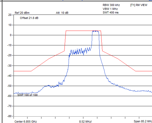
802.11ax (HE20) 52-tone RU : CH 181@40
