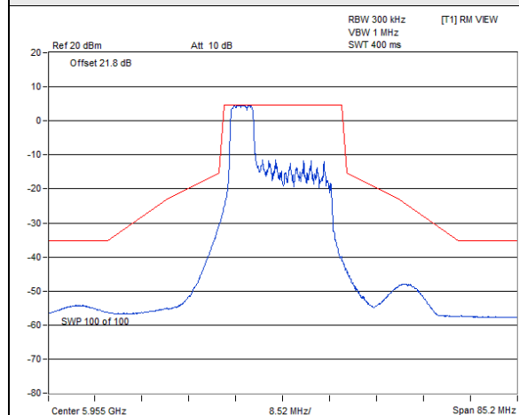
802.11ax (HE20) 52-tone RU : CH 1@37
