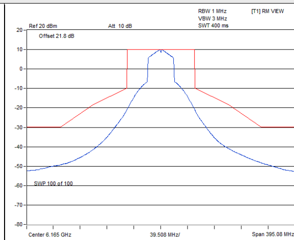
802.11ax (HE40) : CH 43
