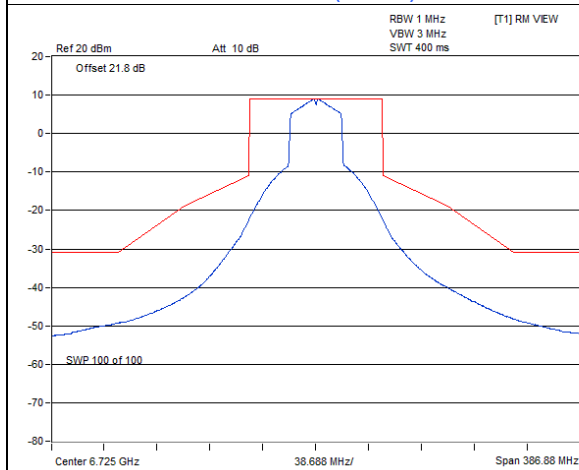
802.11ax (HE40) : CH 155
