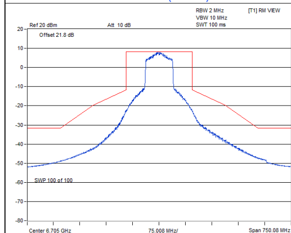
802.11ax (HE80) : CH 151
