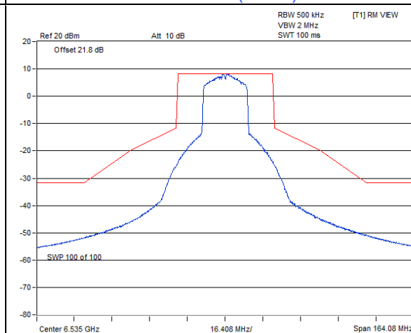
802.11ax (HE20) : CH 117
