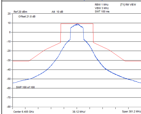
802.11ax (HE40) : CH 91
