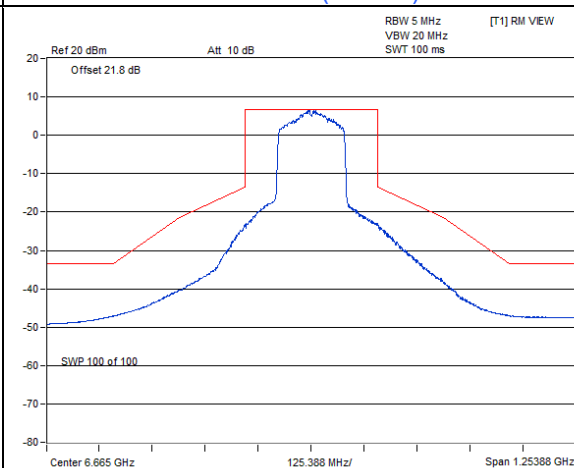
802.11ax (HE160) : CH 143
