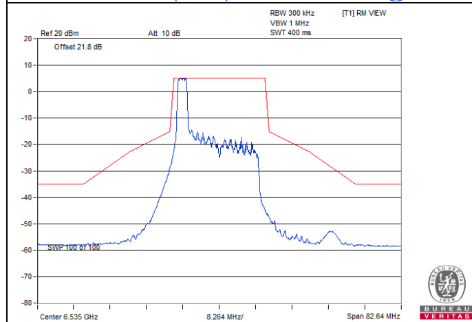
802.11ax (HE20) 26-tone RU : CH 117@0
