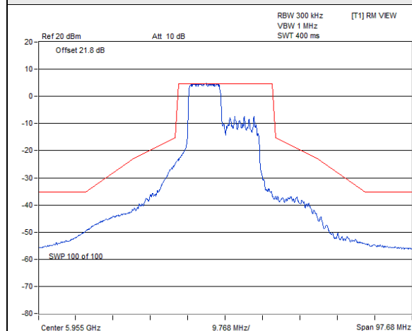
802.11ax (HE20) 106-tone RU : CH 1@53
