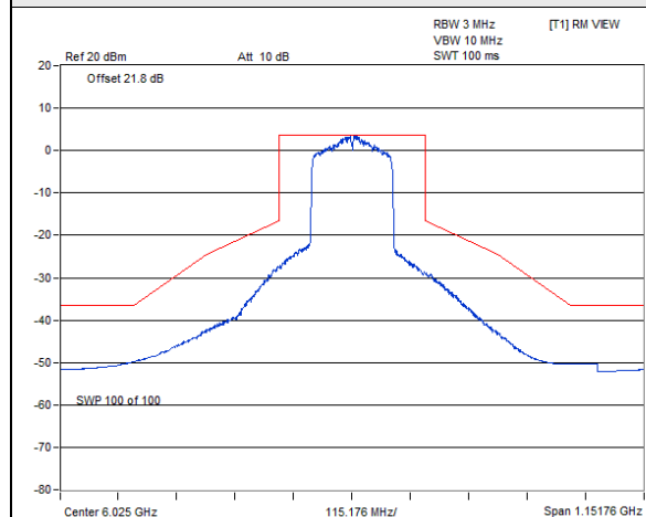
802.11ax (HE160) : CH 15
