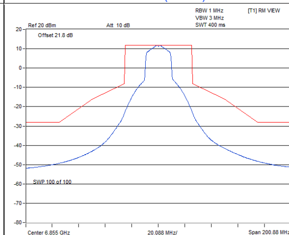
802.11ax (HE20) : CH 181
