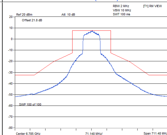
802.11ax (HE80) : CH 167
