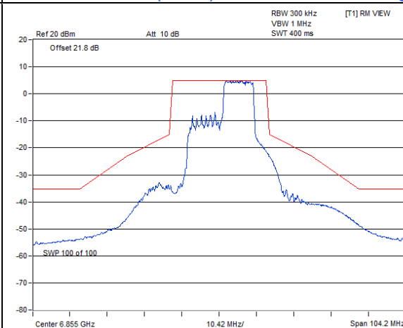
802.11ax (HE20) 106-tone RU : CH 181@54
