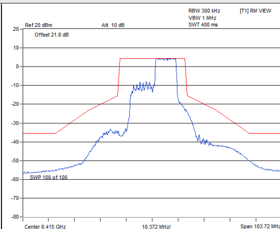
802.11ax (HE20) 106-tone RU : CH 93@54
