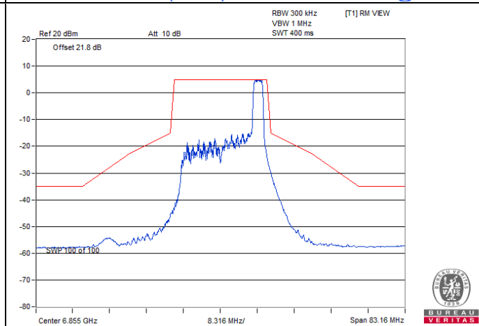
802.11ax (HE20) 26-tone RU : CH 181@8
