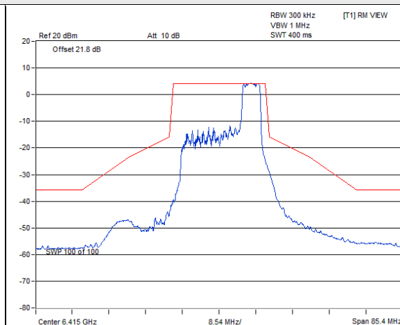
802.11ax (HE20) 52-tone RU : CH 93@40
