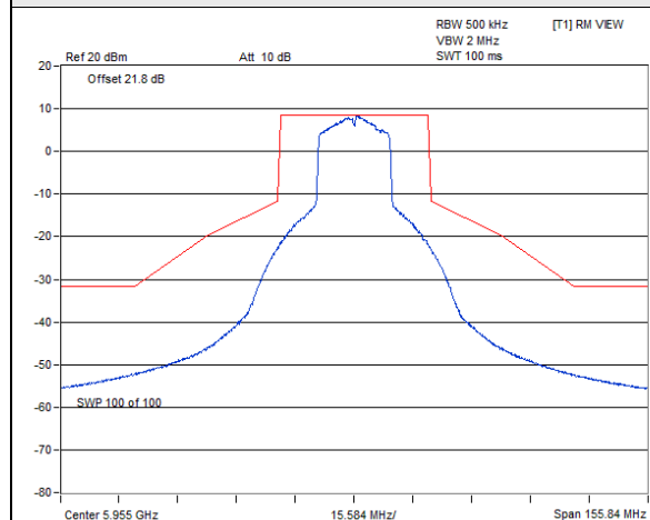
802.11ax (HE20) : CH 1
