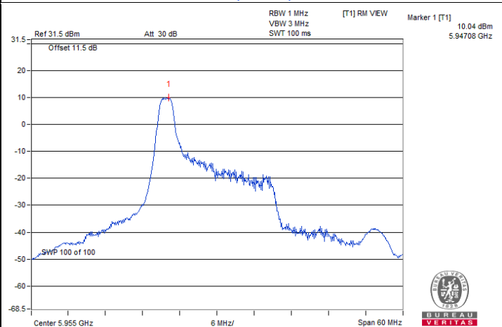
802.11ax (HE20) 26-tone RU : CH 1@0
