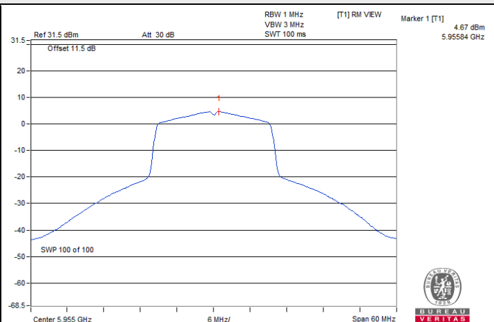
802.11ax (HE20) : CH 1
