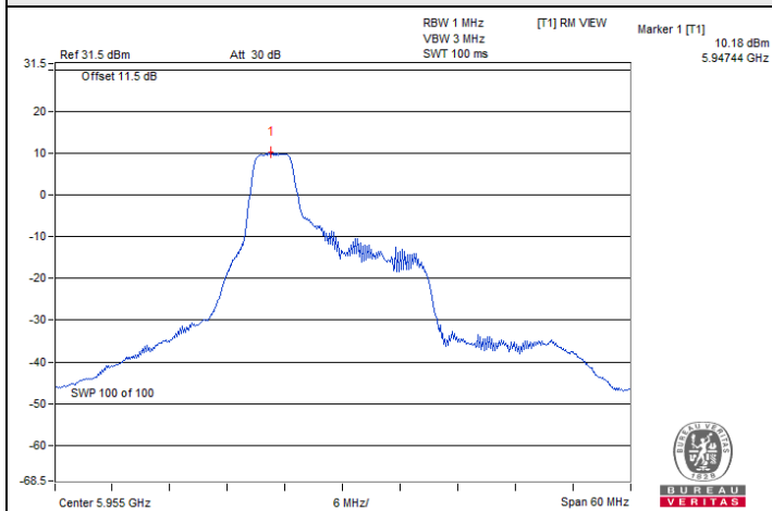
802.11ax (HE20) 52-tone RU : CH 1@37
