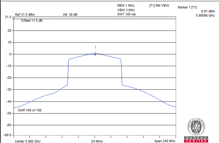
802.11ax (HE80) : CH 7
