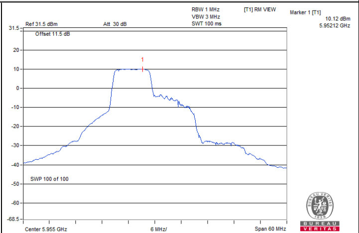
802.11ax (HE20) 106-tone RU : CH 1@53
