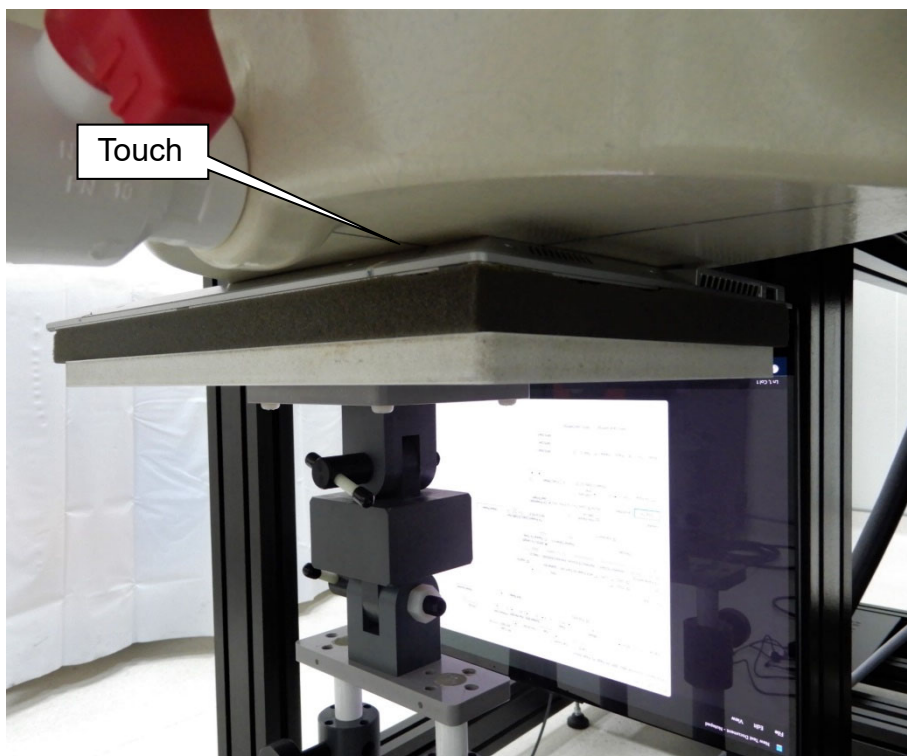
EUT Bottom(NB)_Aux
