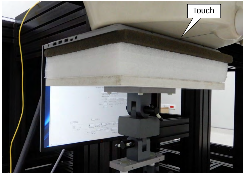
EUT Bottom
