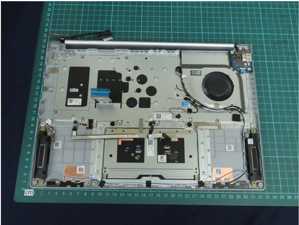
(33) EUT Photo
