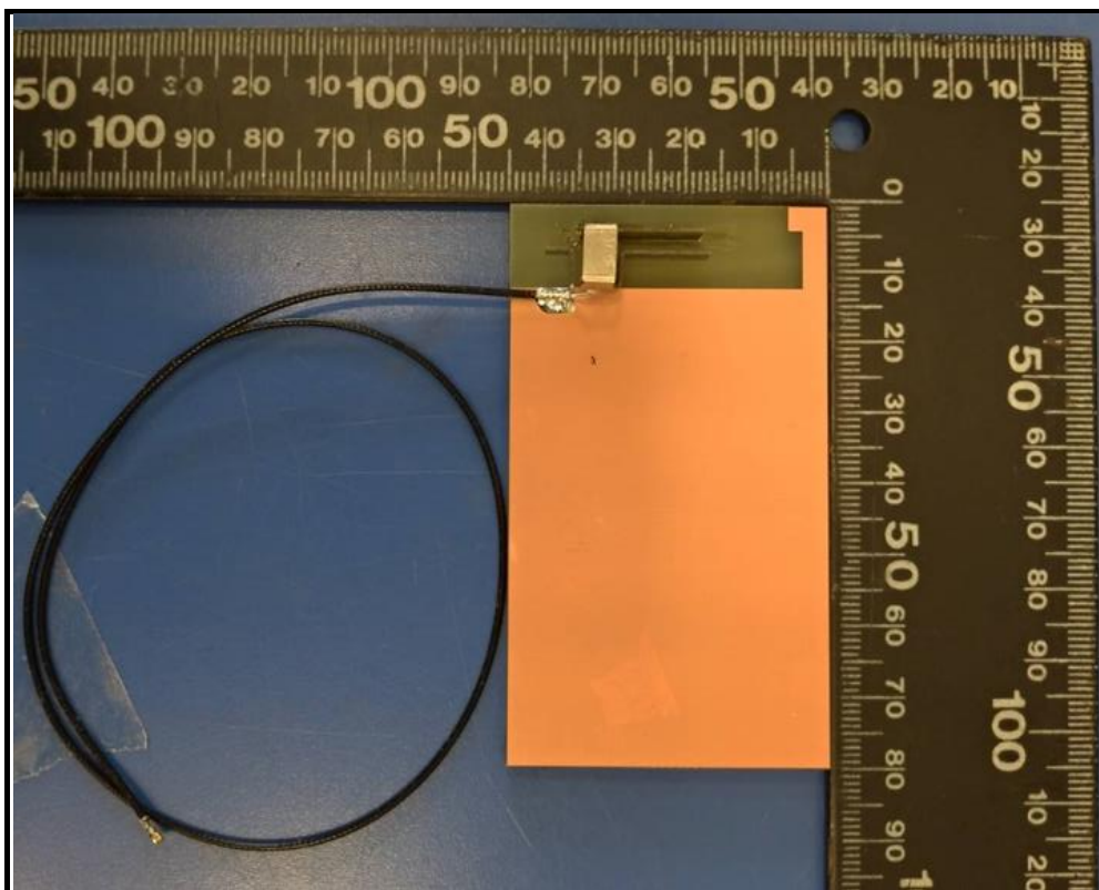
Ant. Set 7 (Brand: HongBo / Model: 260-25106)
