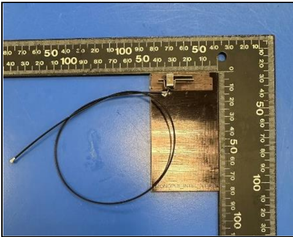
Ant. Set 6 (Brand: HongBo / Model: 260-25105)
