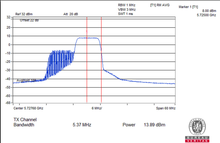
802.11be (EHT20) 106-tone RU 1S1T : CH 144 (U-NII-3)
