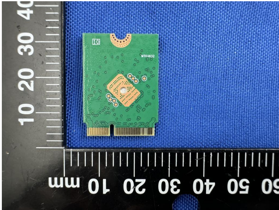
RF MODULE REAR VIEW-MT7925B22M
