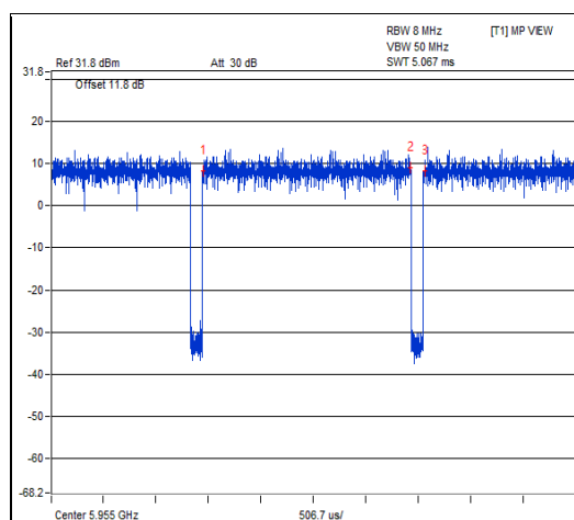
802.11a
