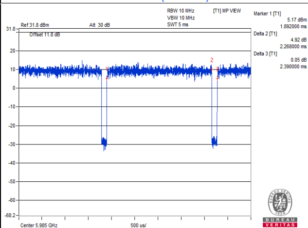
802.11be (EHT80)
