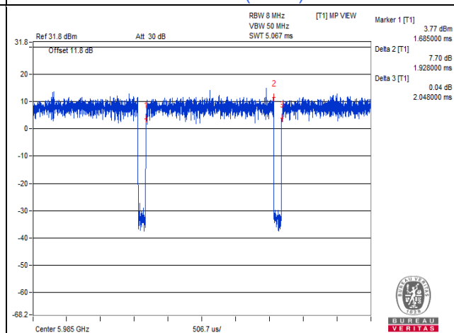
802.11ax (HE80)
