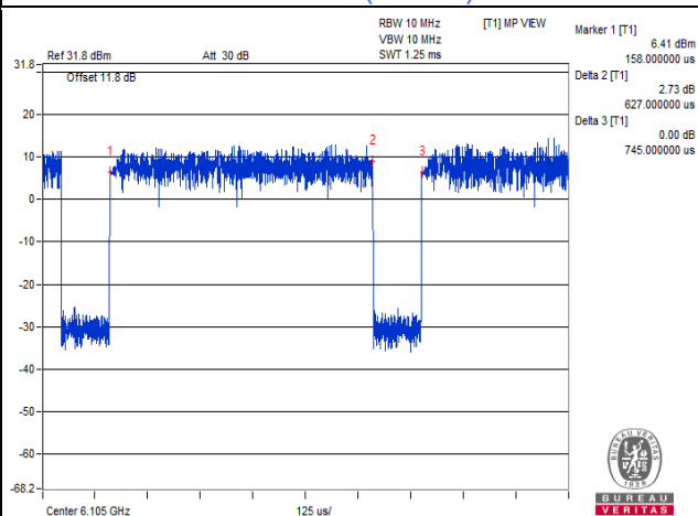
802.11be (EHT320)
