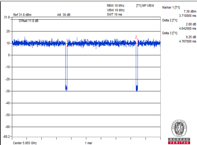
802.11be (EHT20)
