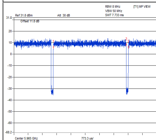
802.11ax (HE40)
