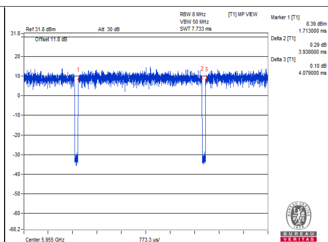
802.11ax (HE20)
