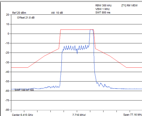
802.11ax (HE) 26-tone RU SP Client_2T2S / Chain 0 : CH 93@8
