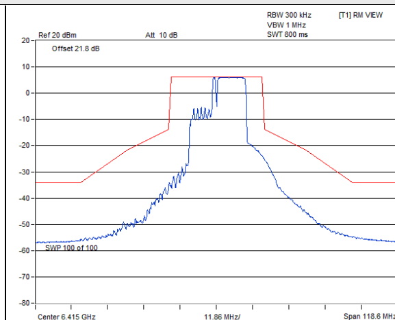
802.11be (EHT20) 106+26-tone MRU SP Client_1T1S : CH 93@83
