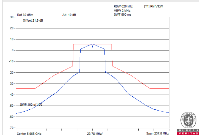
802.11be (EHT40) SP Client 1S1T / Chain 0 : CH 3
