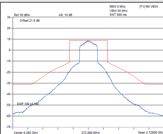
802.11be (EHT320) SP Client 1S1T / Chain 0 : CH 63
