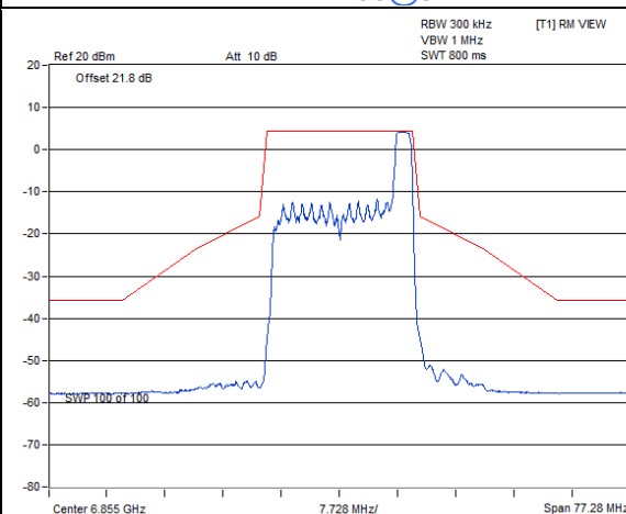
802.11ax (HE) 26-tone RU SP Client_2T2S / Chain 0 : CH 181@8
