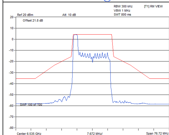
802.11ax (HE) 26-tone RU SP Client_2T2S / Chain 0 : CH 117@0
