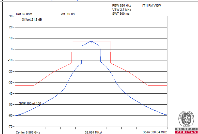
802.11be (EHT40) SP Client 2S2T / Chain 0 : CH 123
