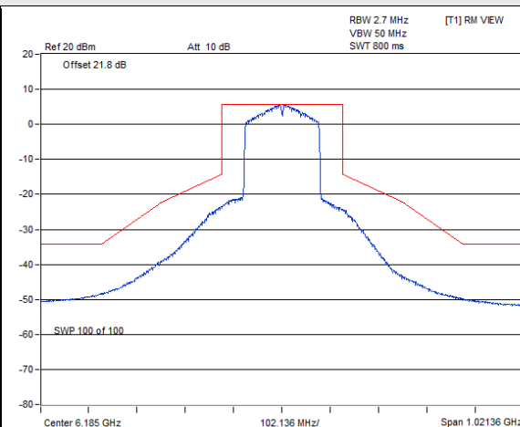
802.11be (EHT160) SP Client 2S2T / Chain 0 : CH 47
