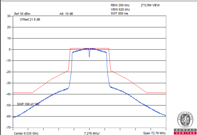
802.11a SP Client 2S2T / Chain 1 : CH 117
