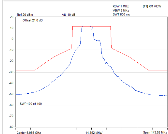
802.11be (EHT20) 106+26-tone MRU SP Client_1T1S : CH 1@82
