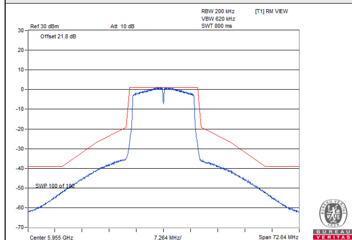
802.11a SP Client 2S2T / Chain 0 : CH 1
