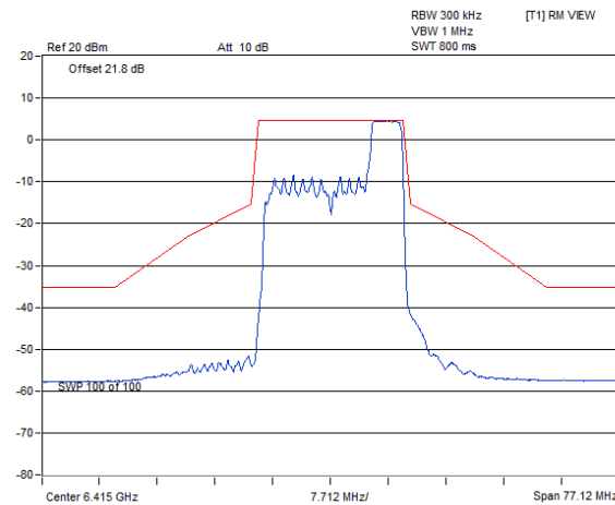
802.11ax (HE) 52-tone RU SP Client_2T2S / Chain 1 : CH 93@40
