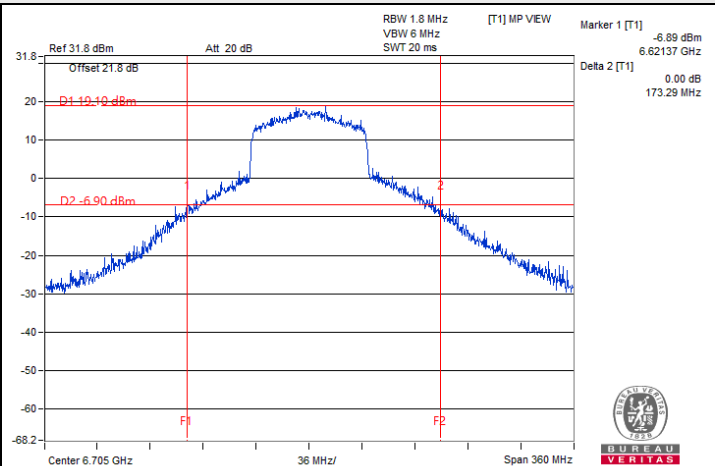
802.11be (EHT80) SP Client 1S1T : CH 151
