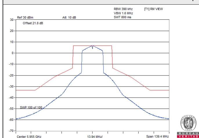
802.11be (EHT20) SP Client 2S2T / Chain 0 : CH 1
