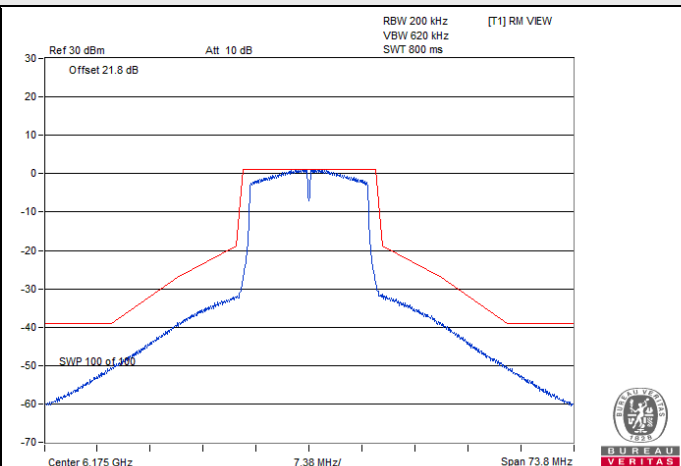
802.11a SP Client 2S2T / Chain 1 : CH 45
