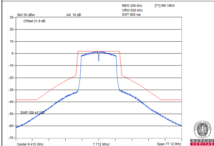
802.11a SP Client 2S2T / Chain 1 : CH 93
