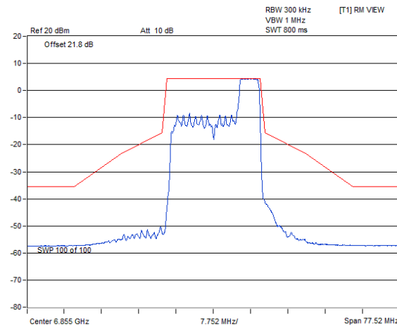
802.11ax (HE) 52-tone RU SP Client_2T2S / Chain 1 : CH 181@40
