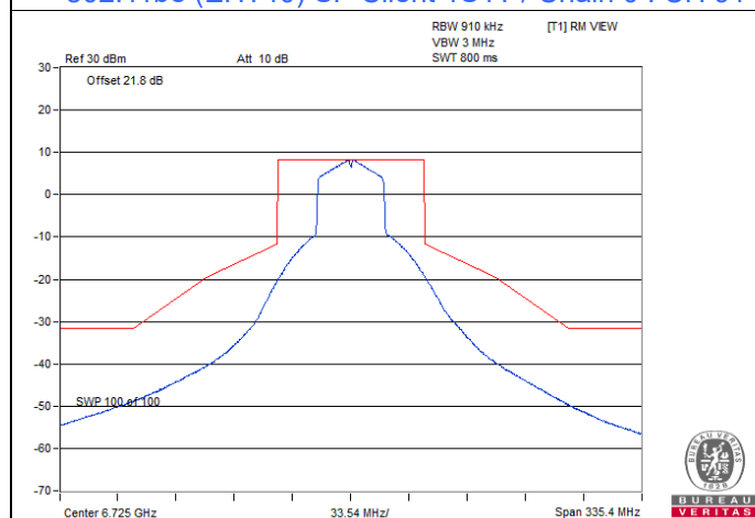
802.11be (EHT40) SP Client 1S1T / Chain 0 : CH 155
