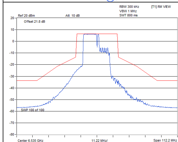
802.11be (EHT20) 106+26-tone MRU SP Client_1T1S : CH 117@82
