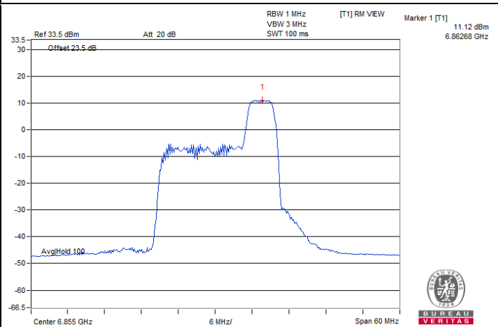
802.11ax (HE) 52-tone RU SP Client_1T1S : CH 181@40
