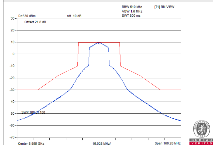
802.11be (EHT20) SP Client 1S1T / Chain 0 : CH 1
