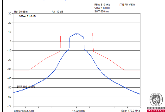
802.11be (EHT20) SP Client 1S1T / Chain 0 : CH 149
