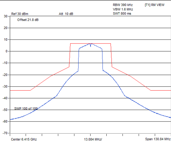
802.11be (EHT20) SP Client 2S2T / Chain 1 : CH 93
