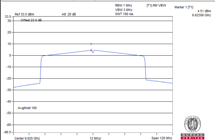
802.11ax (HE80) SP Client 1T1S : CH 135
