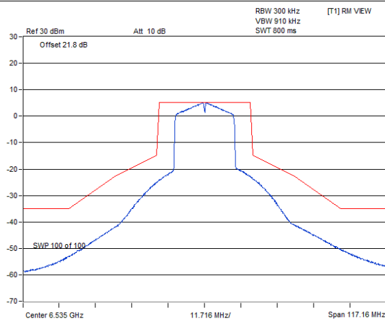
802.11be (EHT20) SP Client 2S2T / Chain 1 : CH 117
