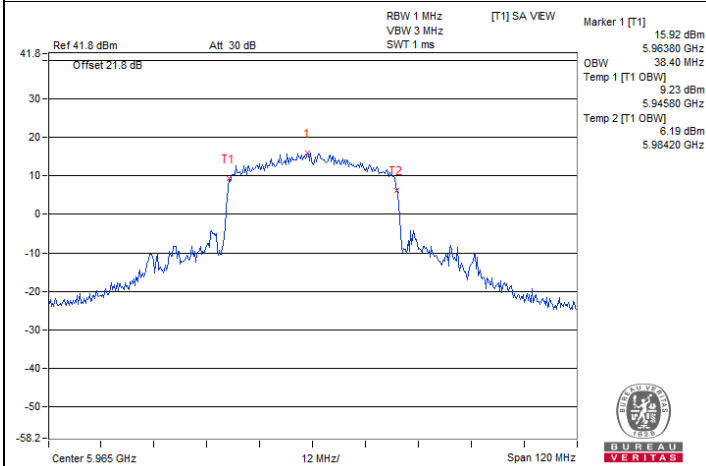
802.11ax (HE40) SP Client 1T1S : CH 3
