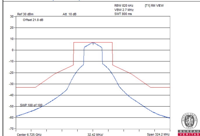
802.11be (EHT40) SP Client 2S2T / Chain 0 : CH 155
