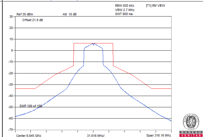
802.11be (EHT40) SP Client 2S2T / Chain 0 : CH 179
