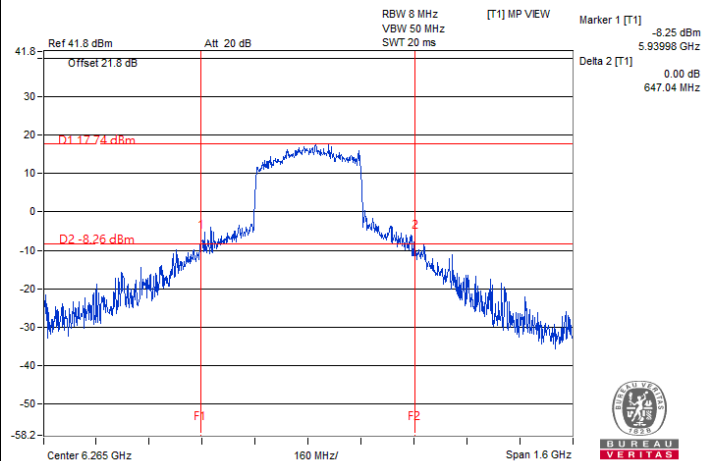
802.11be (EHT320) SP Client 2S2T / Chain 1 : CH 63
