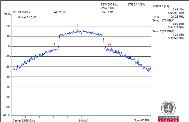
802.11be (EHT20) SP Client 1T1S : CH 1
