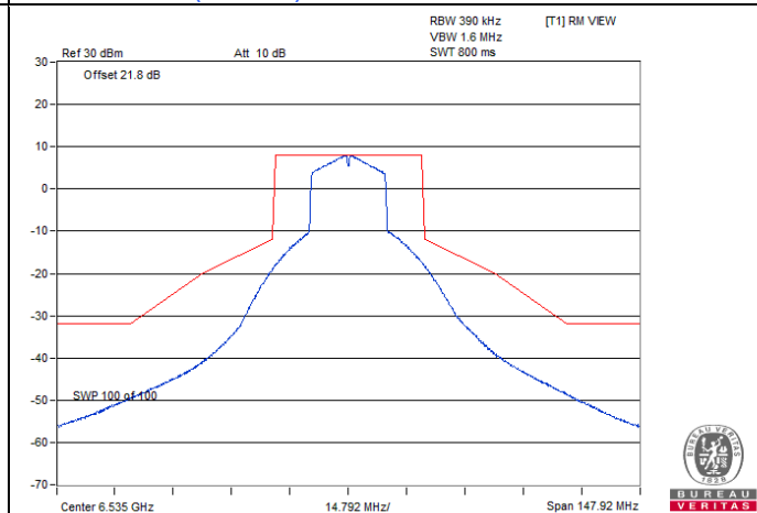
802.11be (EHT20) SP Client 1S1T / Chain 0 : CH 117
