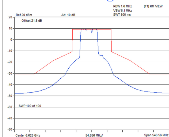
802.11be (EHT80) 484+242-tone MRU SP Client_1T1S : CH 135@93
