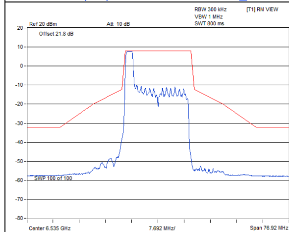
802.11ax (HE) 26-tone RU SP Client_1T1S : CH 117@0
