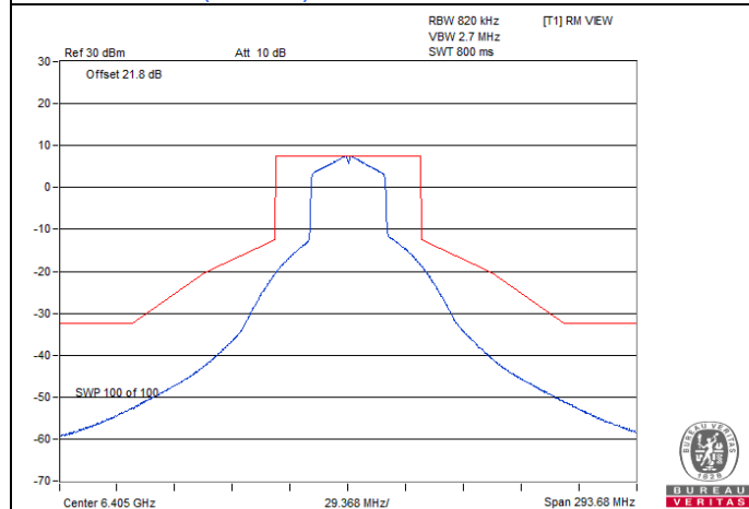
802.11be (EHT40) SP Client 2S2T / Chain 0 : CH 91
