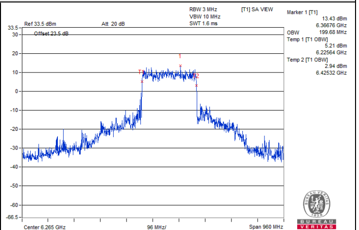
802.11be (EHT320) 2x996+484-tone MRU SP Client 1T1S : CH 63@102_0/1
