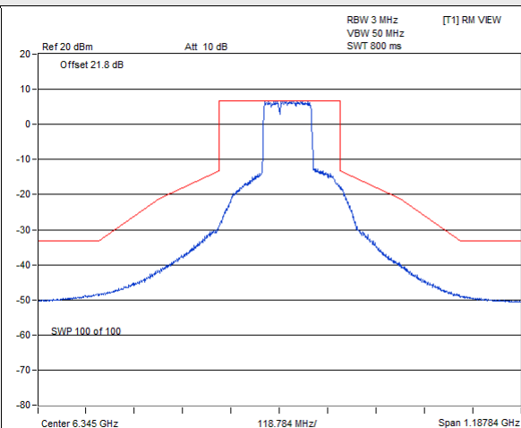
802.11be (EHT160) 996+484-tone MRU SP Client_1T1S : CH 79@94_0
