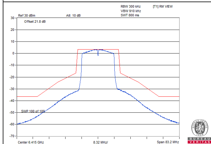
802.11a SP Client 2S2T / Chain 0 : CH 93
