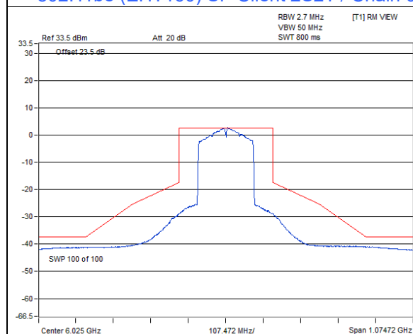
802.11be (EHT160) SP Client 2S2T / Chain 1 : CH 15
