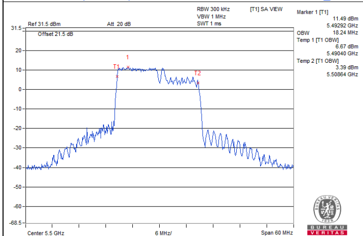
802.11be (EHT20) 106+26-tone MRU / Chain 0 : CH 100@82
