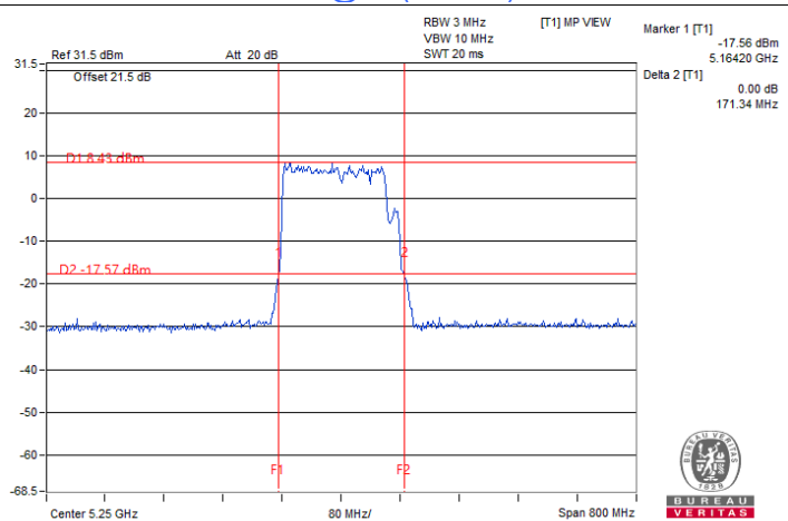
802.11be (EHT160) 996+484+242-tone MRU / Chain 1 : CH 50@99-1 (U-NII-2A)
