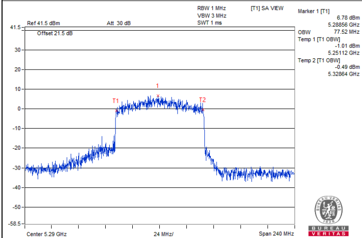
802.11be (EHT80) / Chain 1 : CH 58
