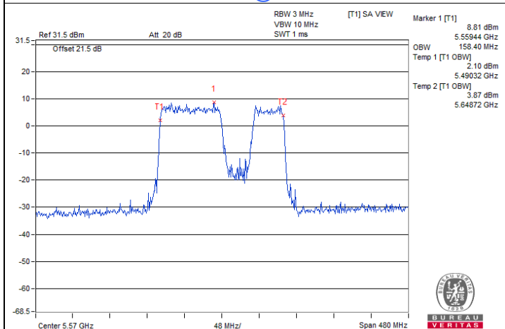
802.11be (EHT160) 996+484-tone MRU / Chain 0 : CH 114@94-1
