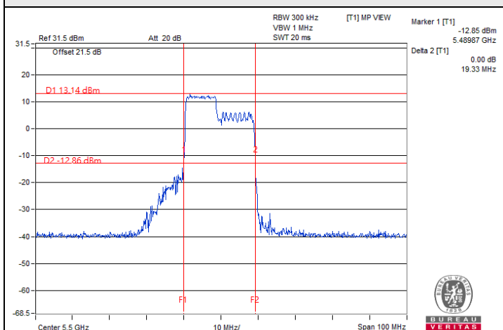
802.11be (EHT20) 106-tone RU / Chain 0 : CH 100@53
