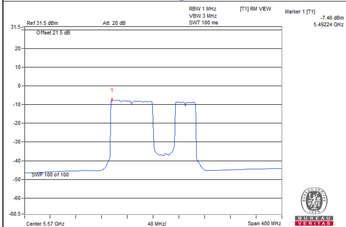
802.11be (EHT160) 996+484-tone MRU / Chain 1 : CH 114@94-1
