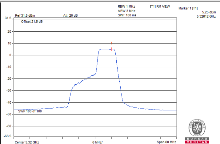
802.11be (EHT20) 52+26-tone MRU / Chain 0 : CH 64@72
