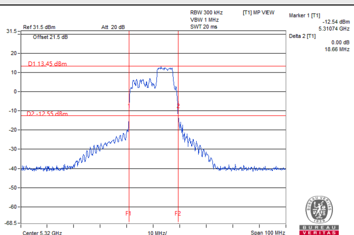
802.11be (EHT20) 52+26-tone MRU / Chain 1 : CH 64@72
