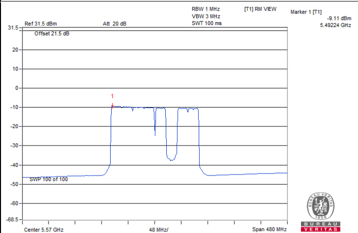
802.11be (EHT160) 996+484+242-tone MRU / Chain 1 : CH 114@97-1
