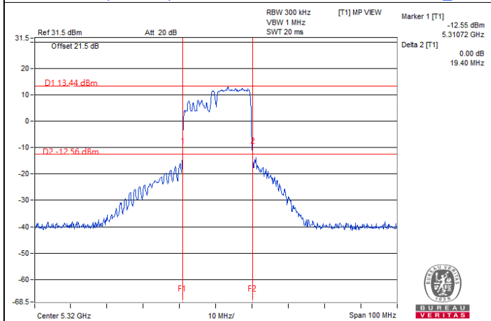
802.11be (EHT20) 106+26-tone MRU / Chain 1 : CH 64@83
