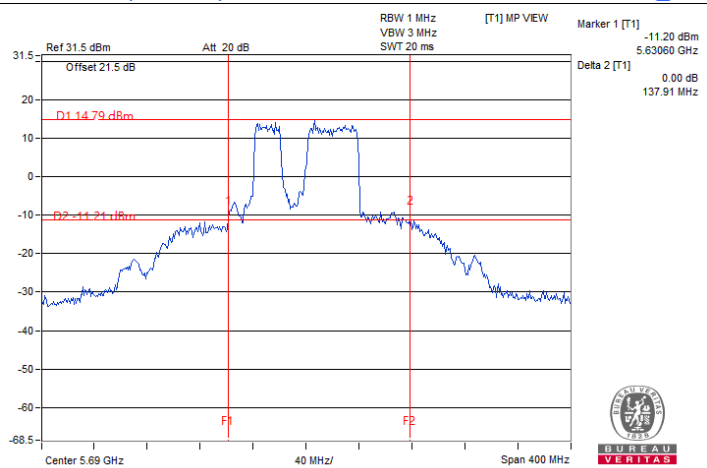
802.11be (EHT80) 484+242-tone MRU / Chain 0 : CH 138@91 (U-NII-3)
