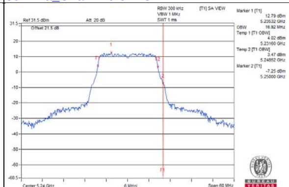
802.11a_Chain 3 / CH48
