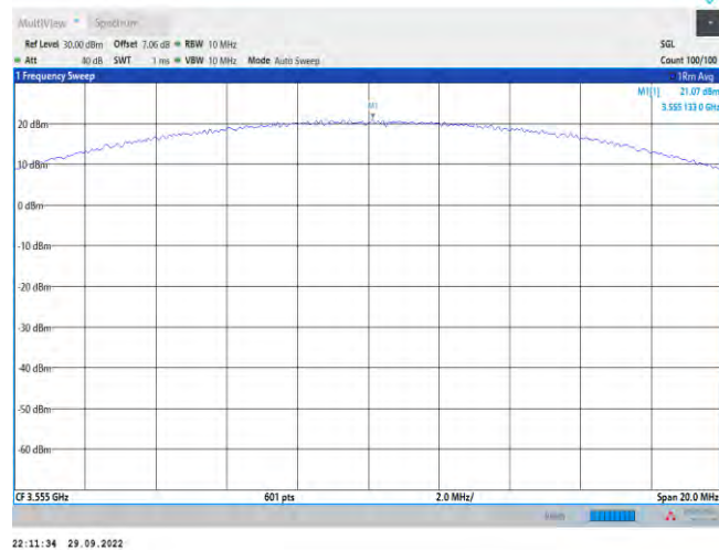
Band48-10MHz-QPSK-55290-1RB#24
