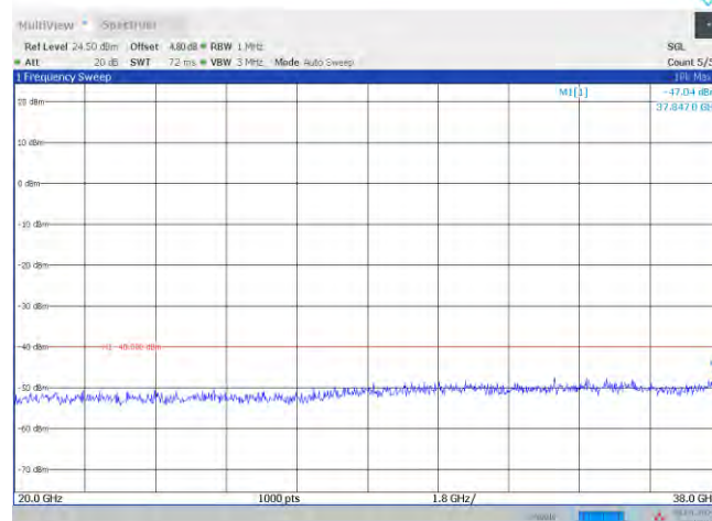
Band48-20MHz-QPSK-55990-1RB#0-Range5:20000~38000MHz
