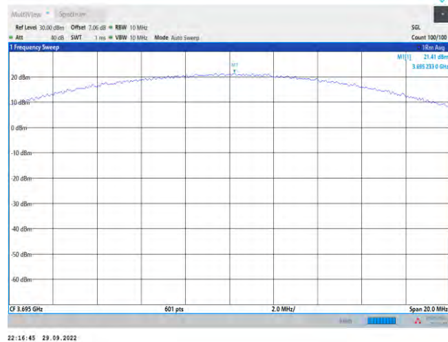
Band48-10MHz-QPSK-56690-1RB#24
