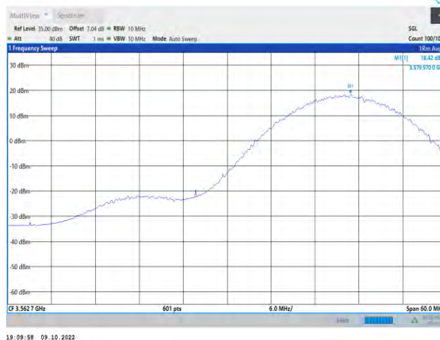
48-48-10MHz-20MHz-QPSK-QPSK-55295-55439-1RB#0-0RB#0
