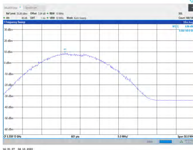
48-48-5MHz-20MHz-QPSK-QPSK-55273-55390-1RB#0-0RB#0
