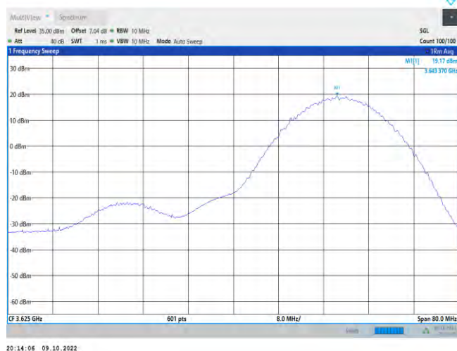
48-48-20MHz-20MHz-QPSK-QPSK-55891-56089-100RB#0-100RB#0
