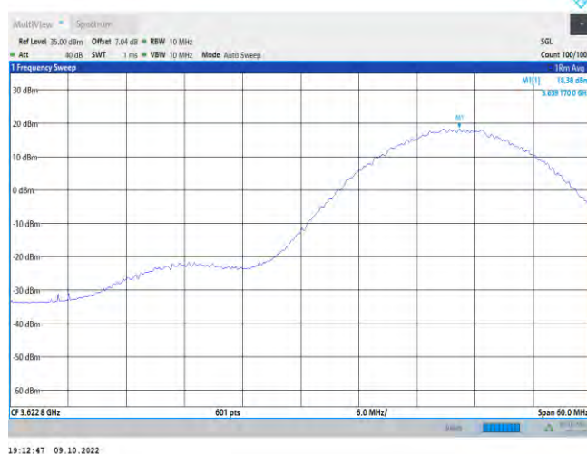
48-48-10MHz-20MHz-QPSK-QPSK-55896-56040-1RB#0-ORB#0
