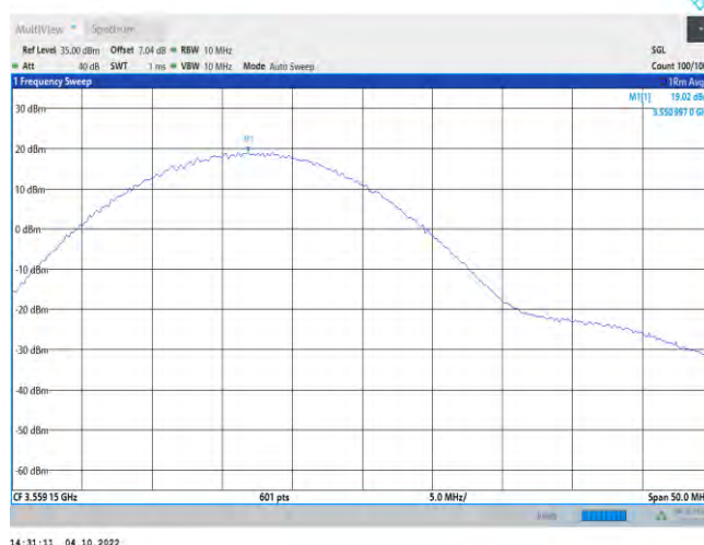
48-48-5MHz-20MHz-QPSK-QPSK-55273-55390-25RB#0-100RB#0
